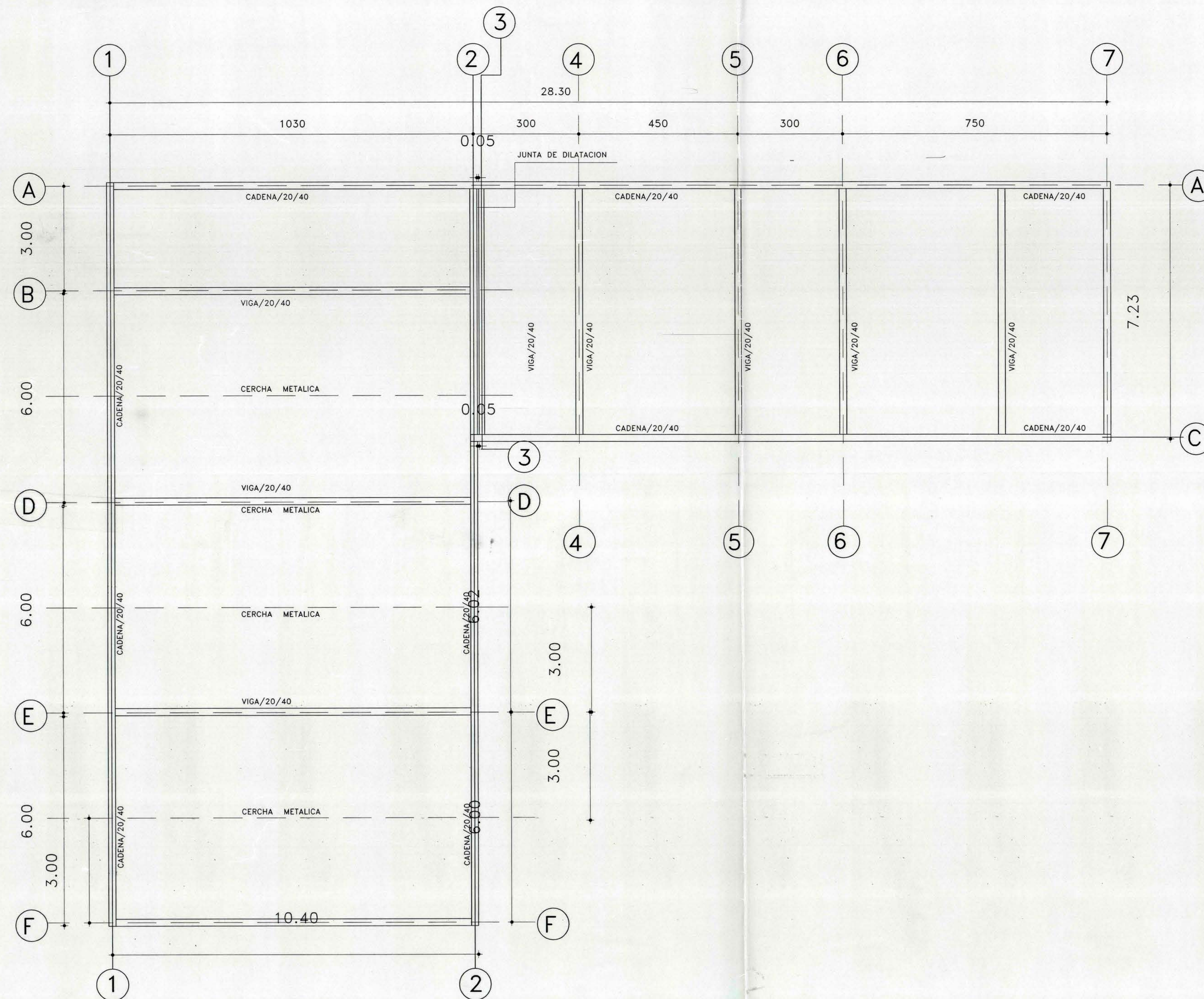
PLANTA DE ESTRUCTURAS ESC. 1:50
