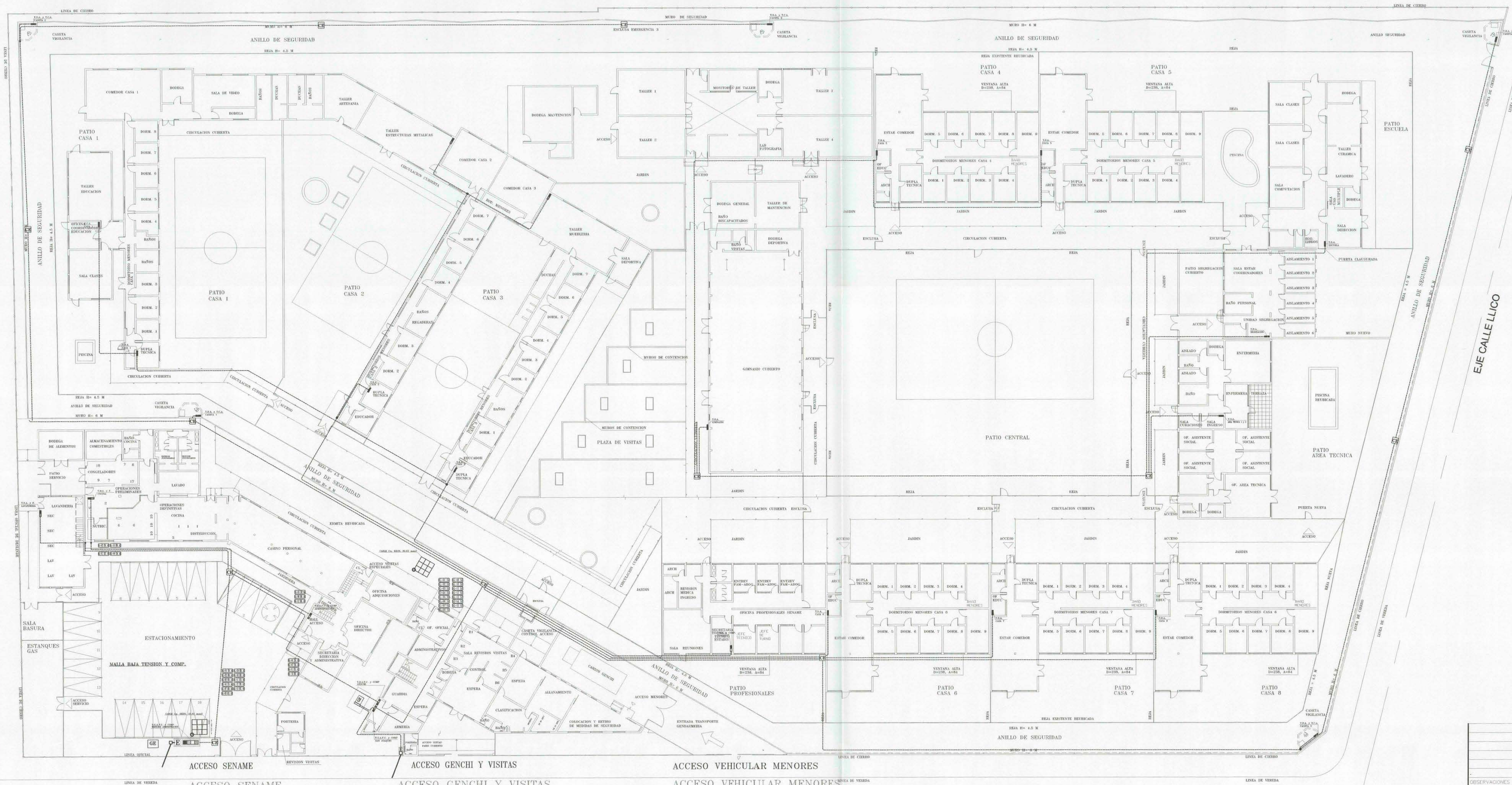
PLANTA PRIMER PISO ESC. 1/200
