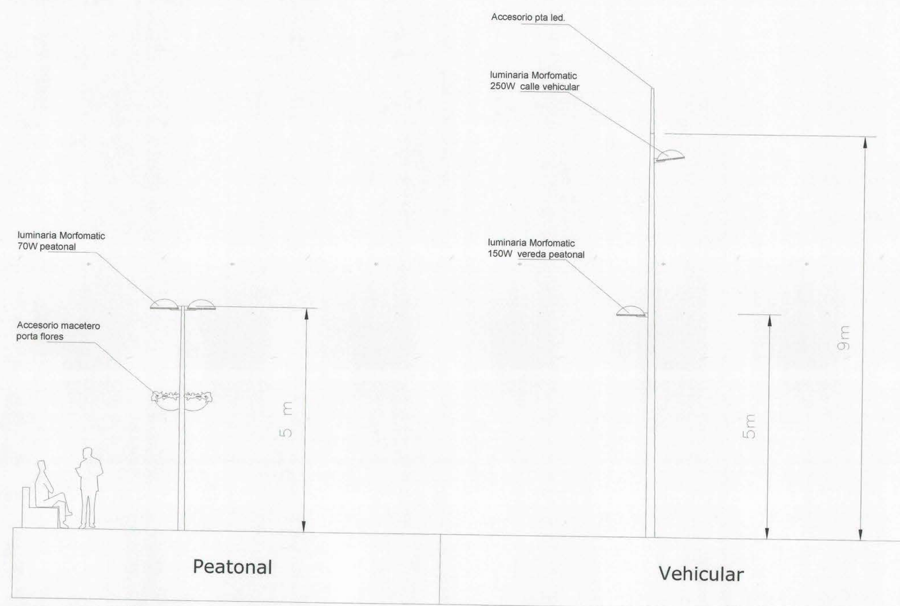
ESQUEMÁTICO ESC 1:50
