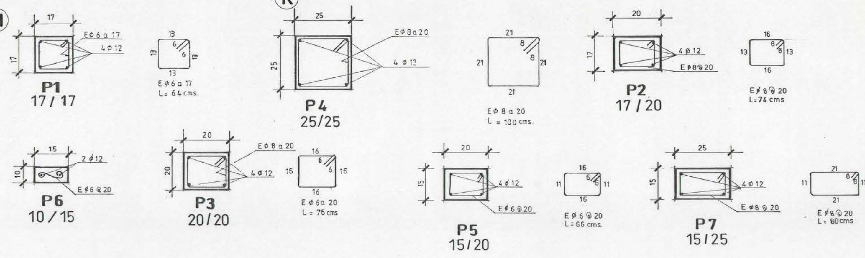
DETALLE DE PILARES ESCALA 1:10
