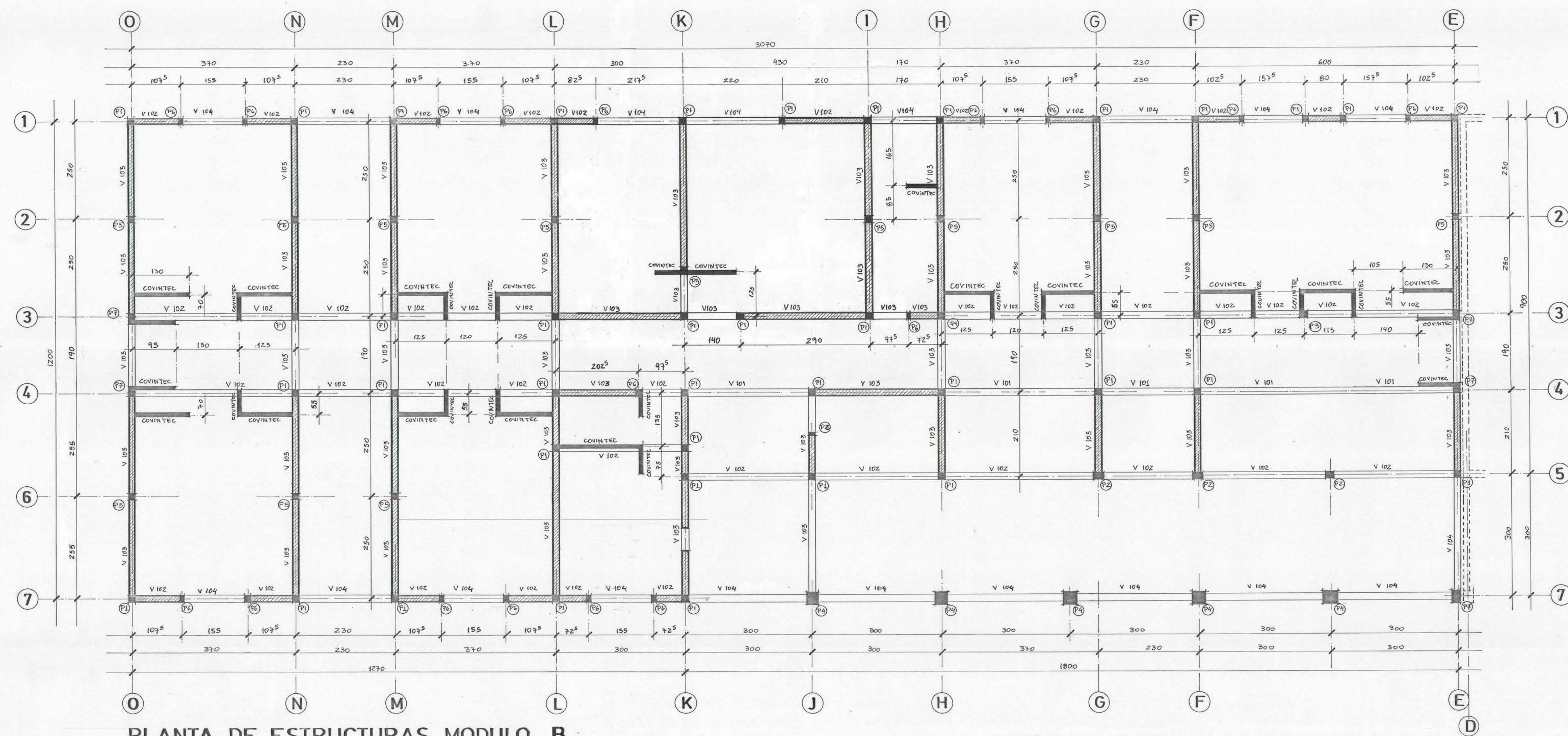
PLANTA DE ESTRUCTURAS MODULO B
