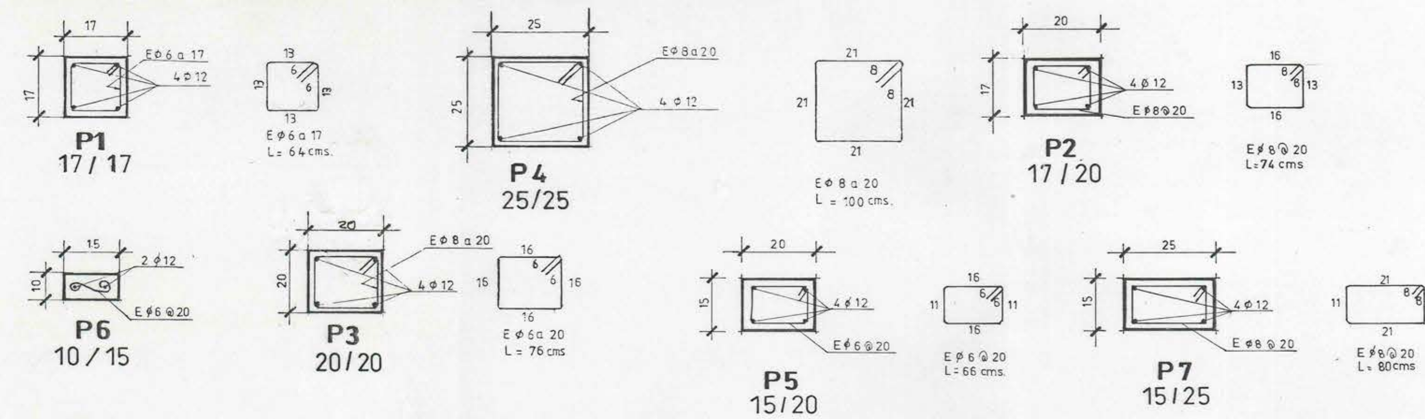
DETALLE DE PILARES ESCALA 1:10
