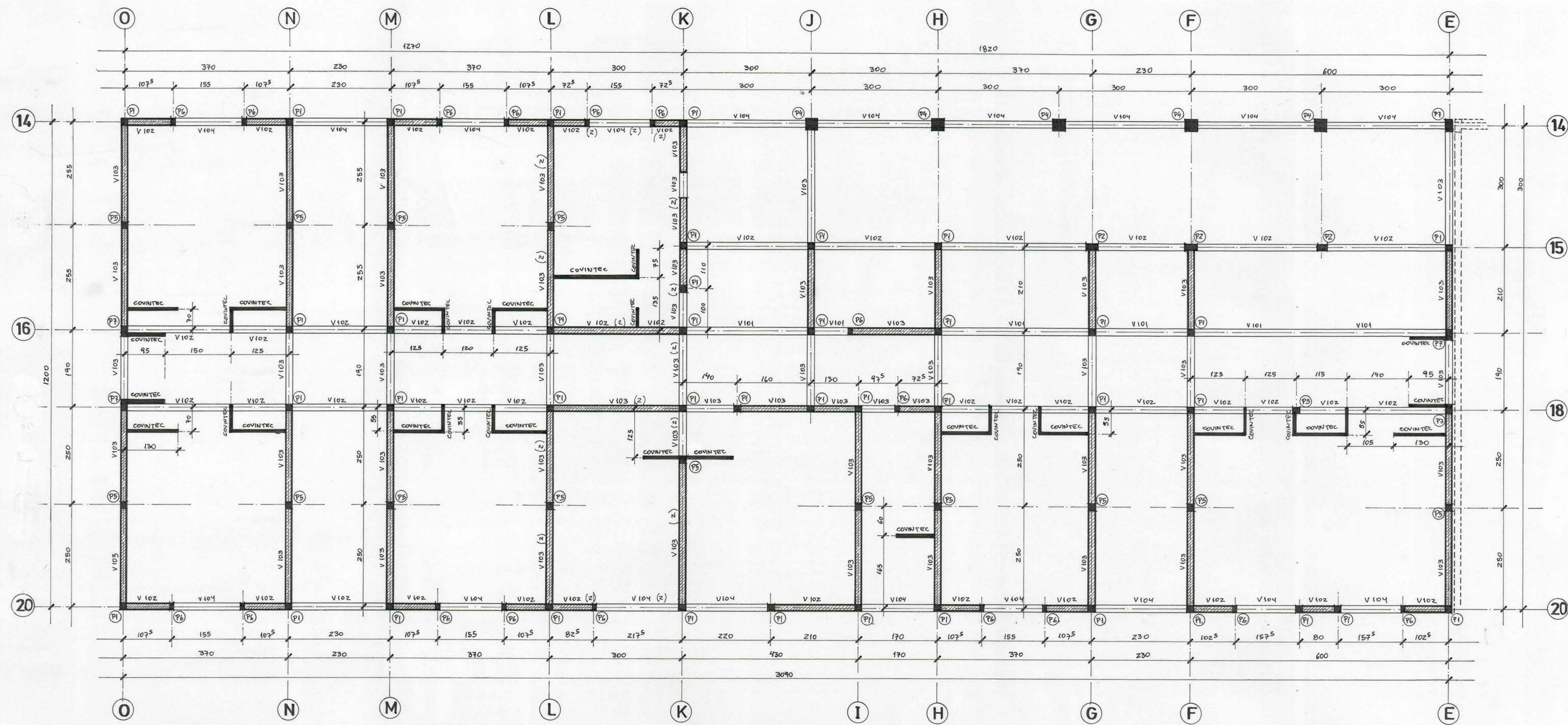
PLANTA DE ESTRUCTURAS MODULO C
