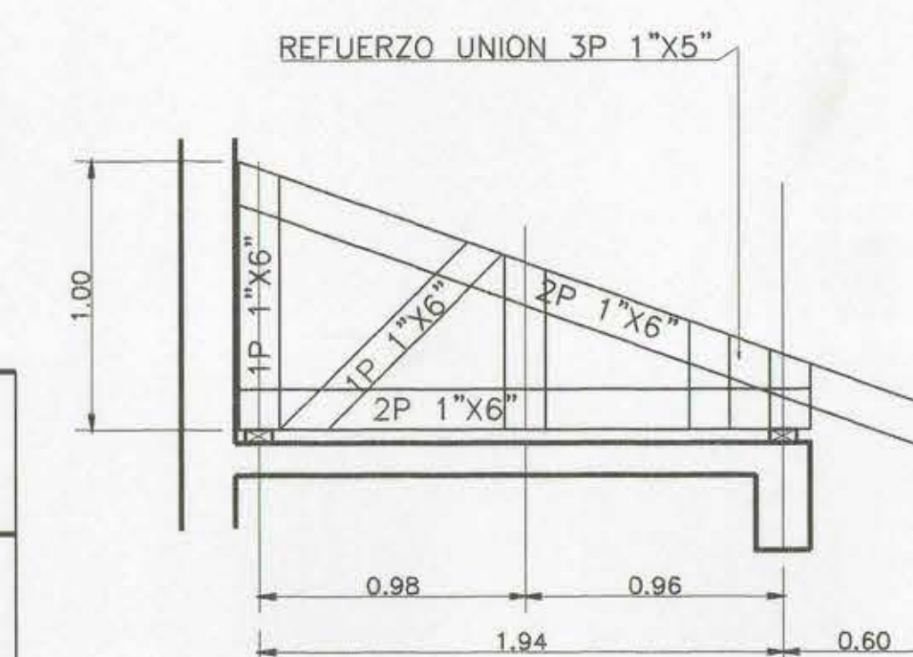
CERCHA C2 ESCALA 1:25
