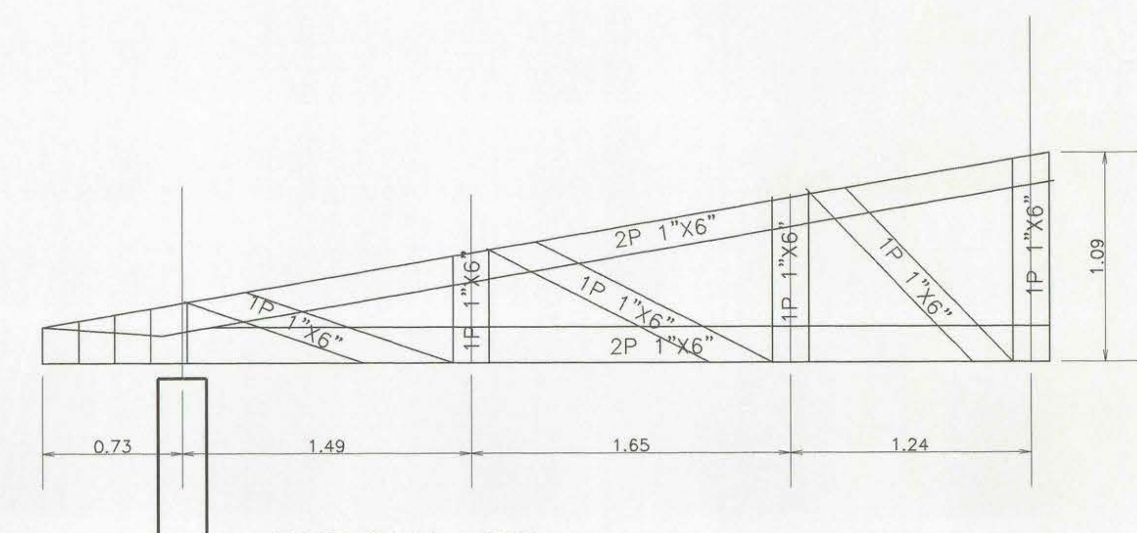
CERCHA C3 ESCALA 1:20
