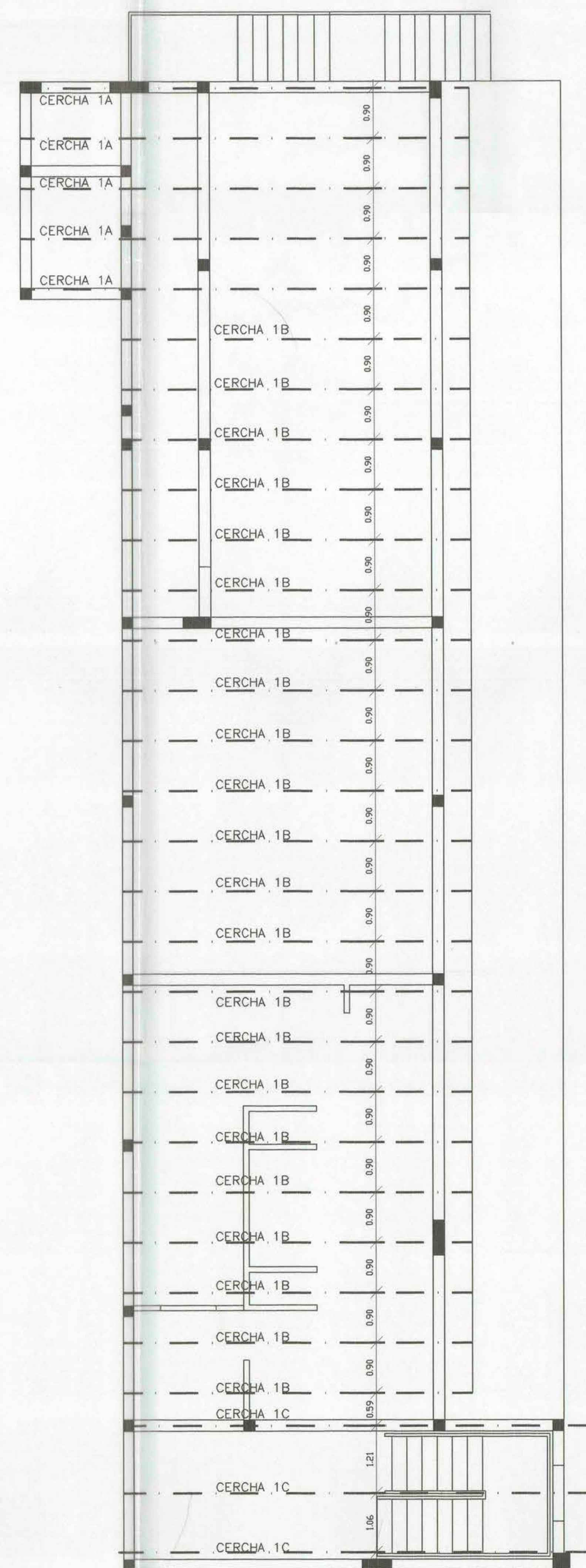
PLANTA ESTRUCTURAS TECHUMBRE SEGUNDO PISO ESCALA 1:100
