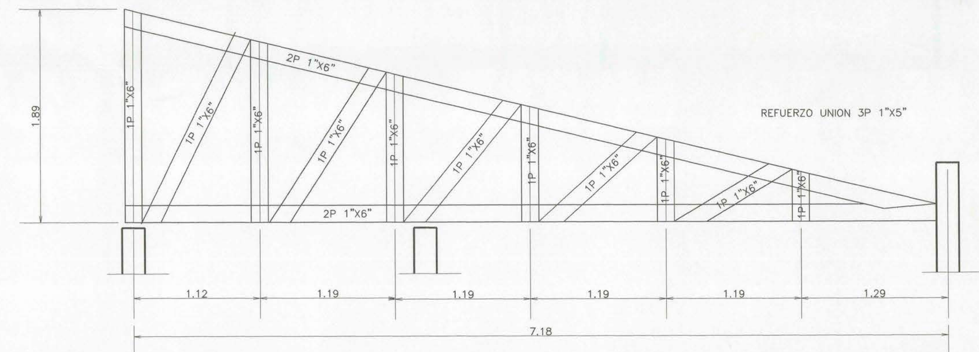
CERCHA C5 ESCALA 1:20
