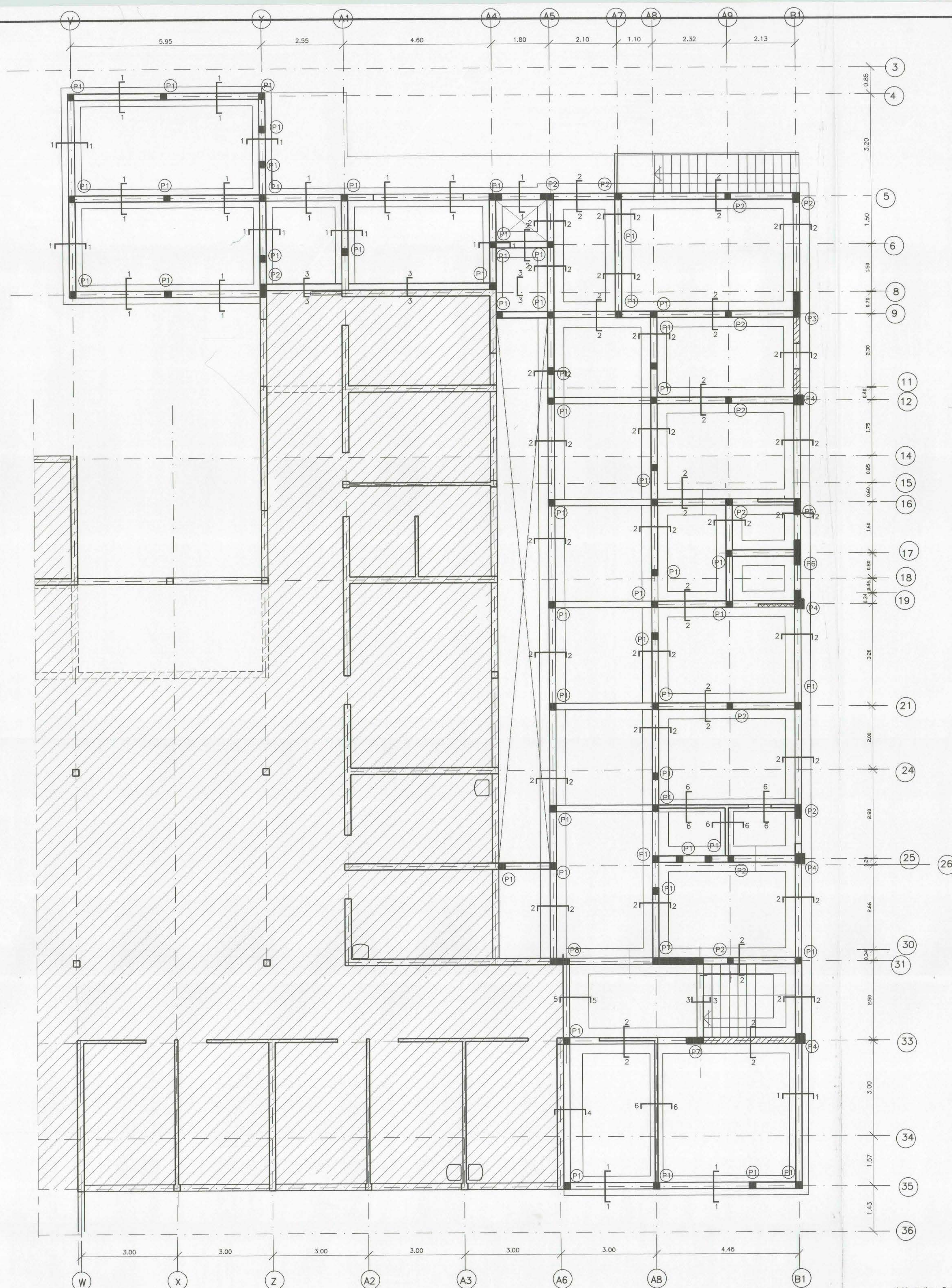
PLANTA FUNDACIONES MOD. A ESCALA 1 : 100
