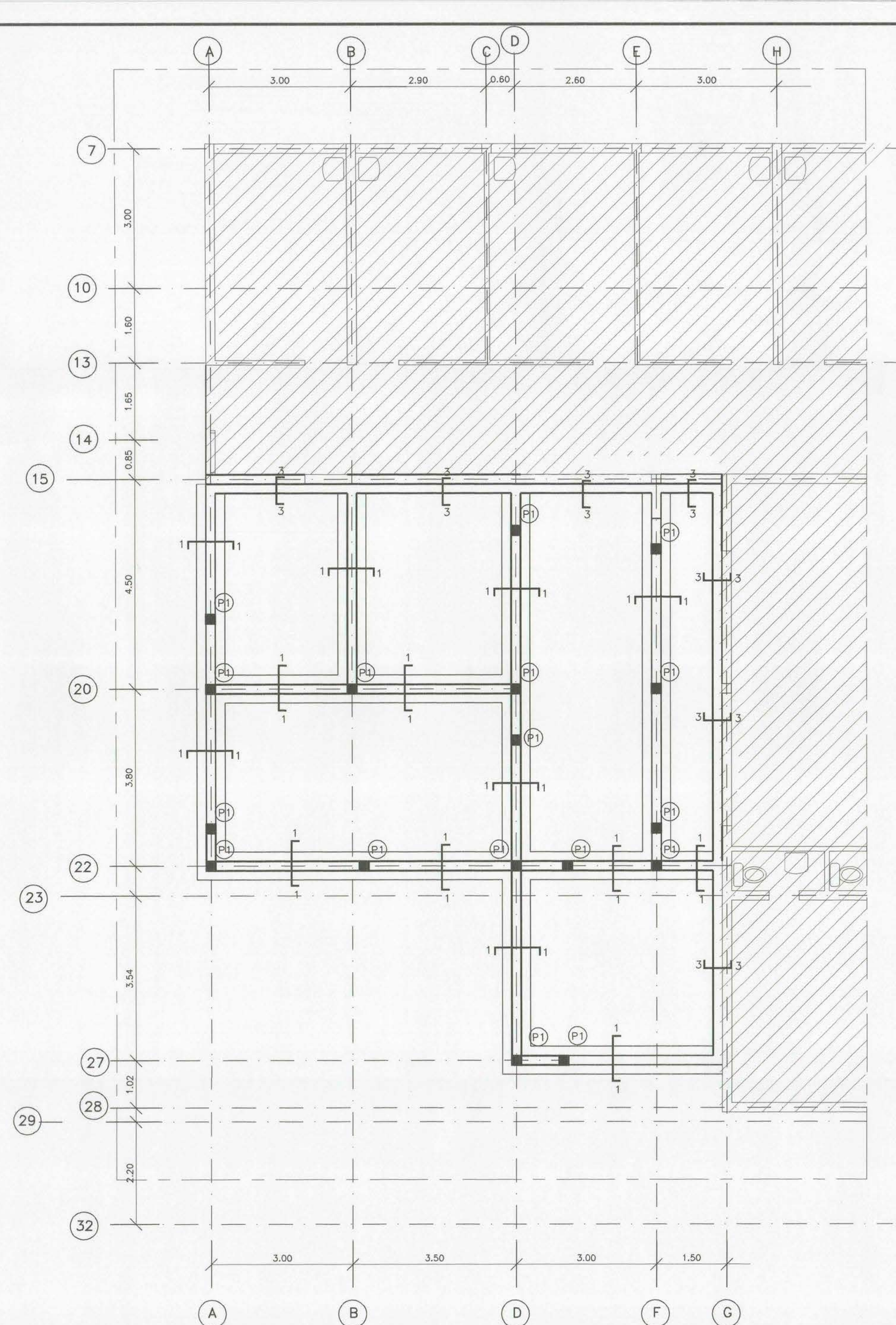
PLANTA FUNDACIONES MODULO C ESCALA 1 : 100
