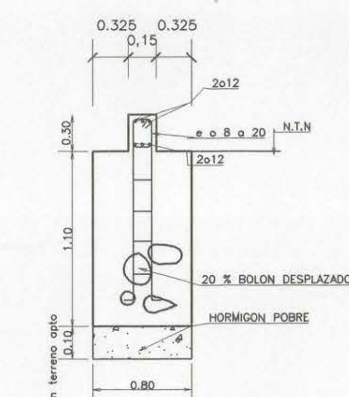
CORTE 2-2 VIGA FUNDACION
