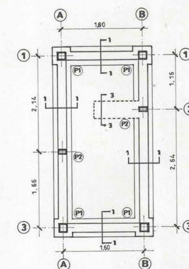
PLANTA FUNDACIONES ESCALA 1:50
