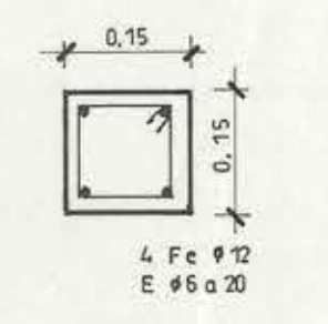
PILAR P1 15/15 ESCALA 1:10
