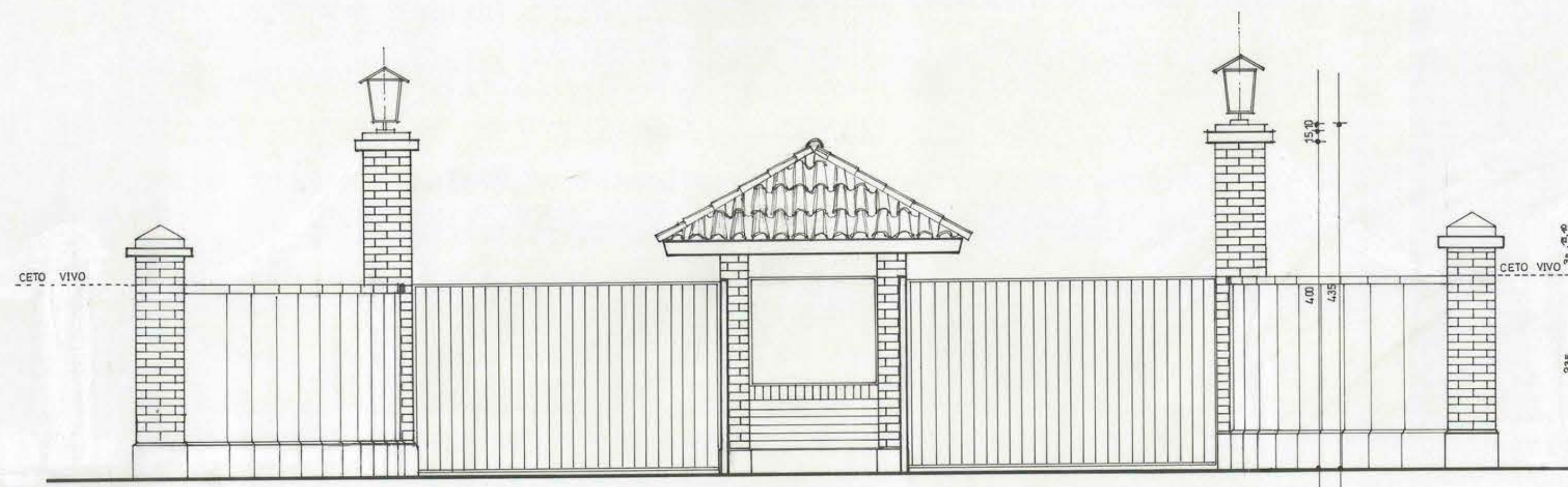
ELEVACION ESC. 1/50 ACCESO TIPO (son 2)
