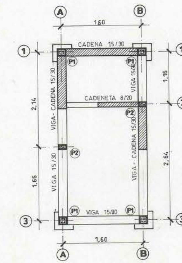
PLANTA ESTRUCTURAS PLANTA 1:50
