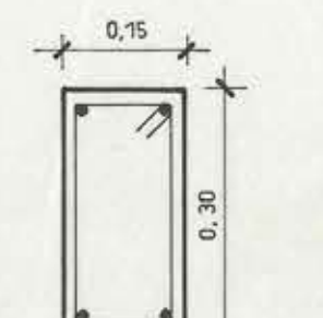
E 66a20 VIGA - CADENA 15/30 ESCALA 1:10
