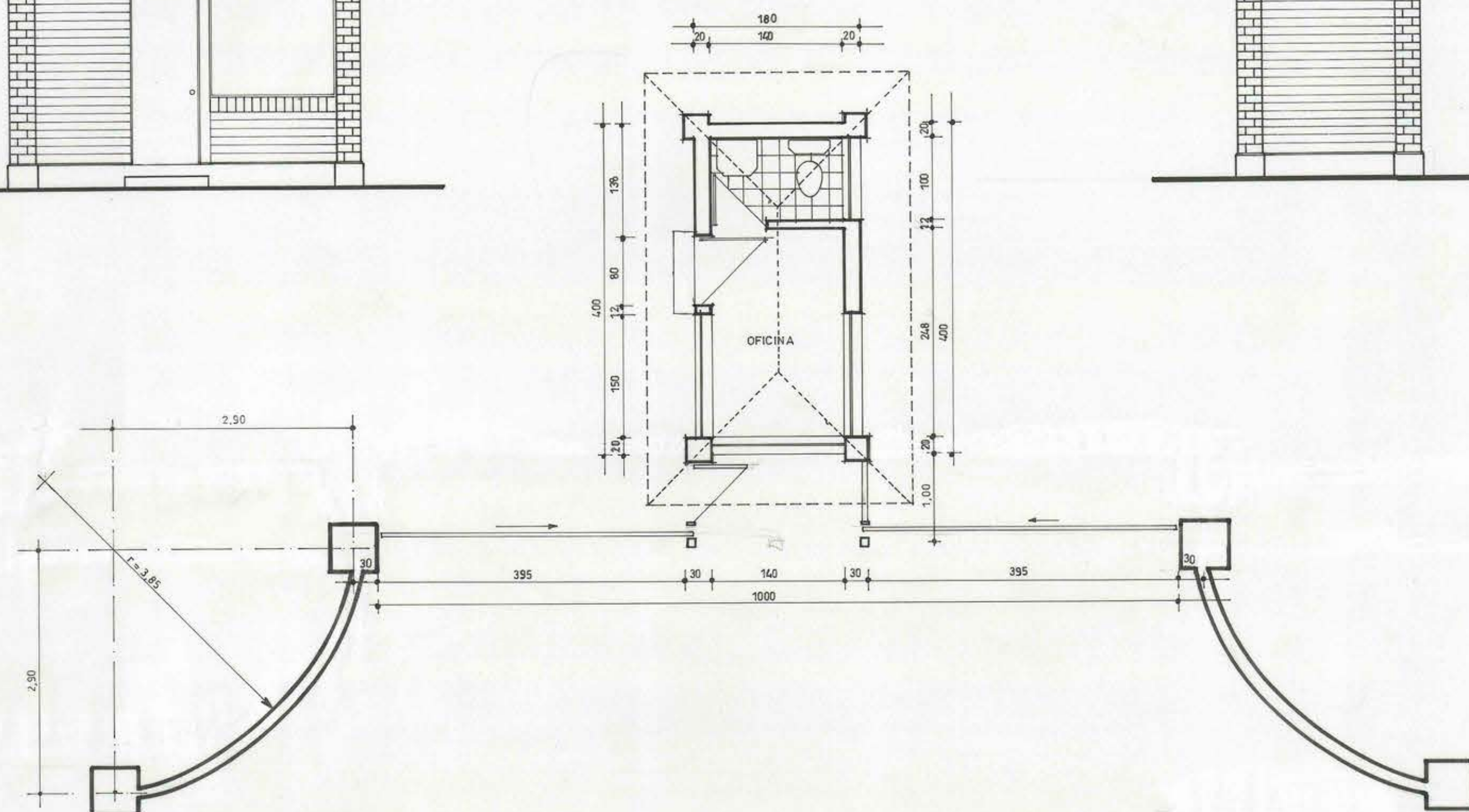
PLANTA ESCALA 1:50
