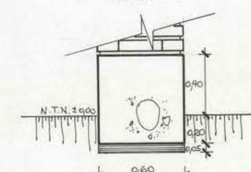
CORTE POYO FUNDACION 2-2 ESCALA 1:25
