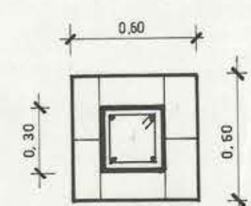
PILAR P3 30/30 4 Fe Ø 12 E Ø 60 20
