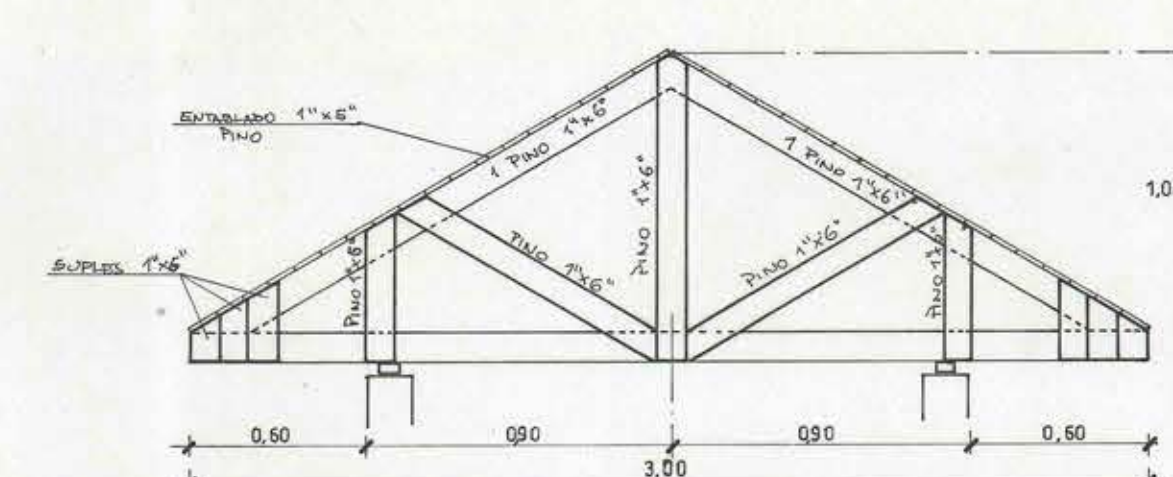
CERCHA C1 ESCALA 1:25
