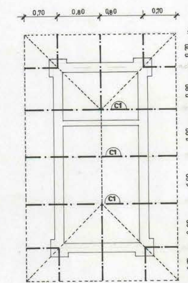
PLANTA TECHUMBRE PLANTA 1:50
