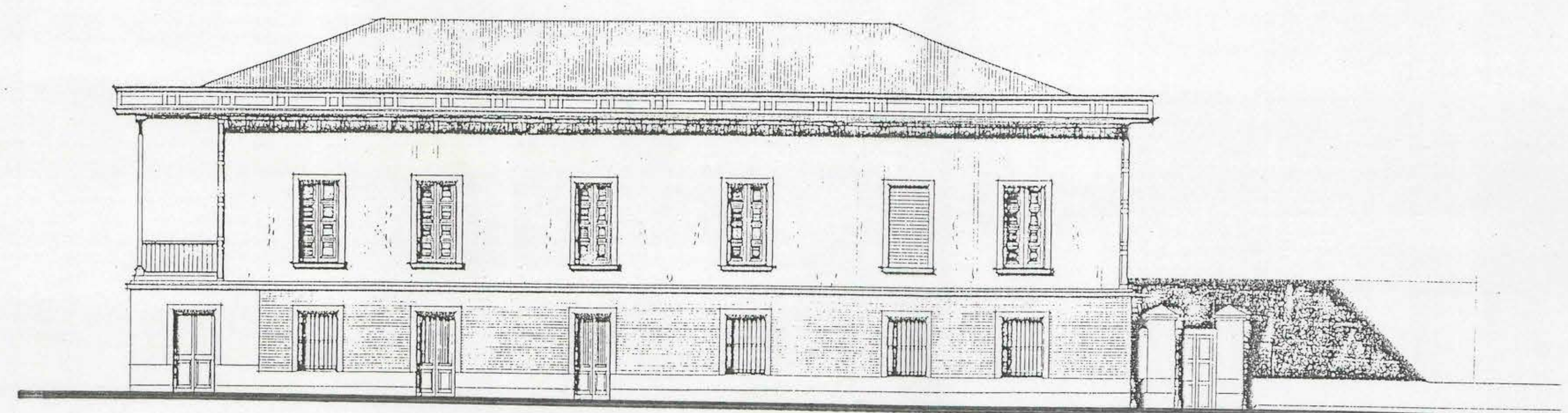
FACHADA PONIENTE CALLE O'HIGGINS 1:100
