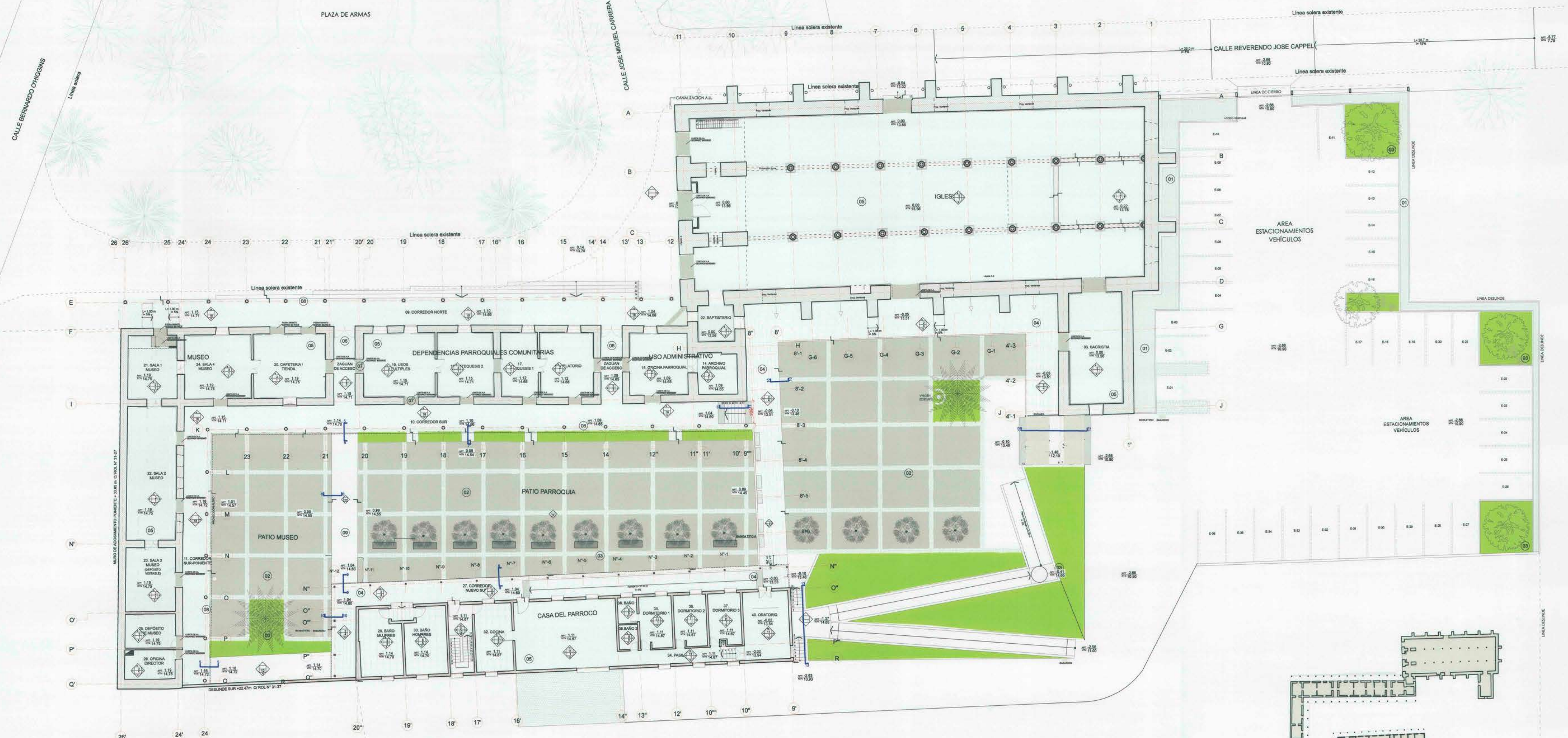
PLANTA GENERAL PAVIMENTOS ESC 1:200
