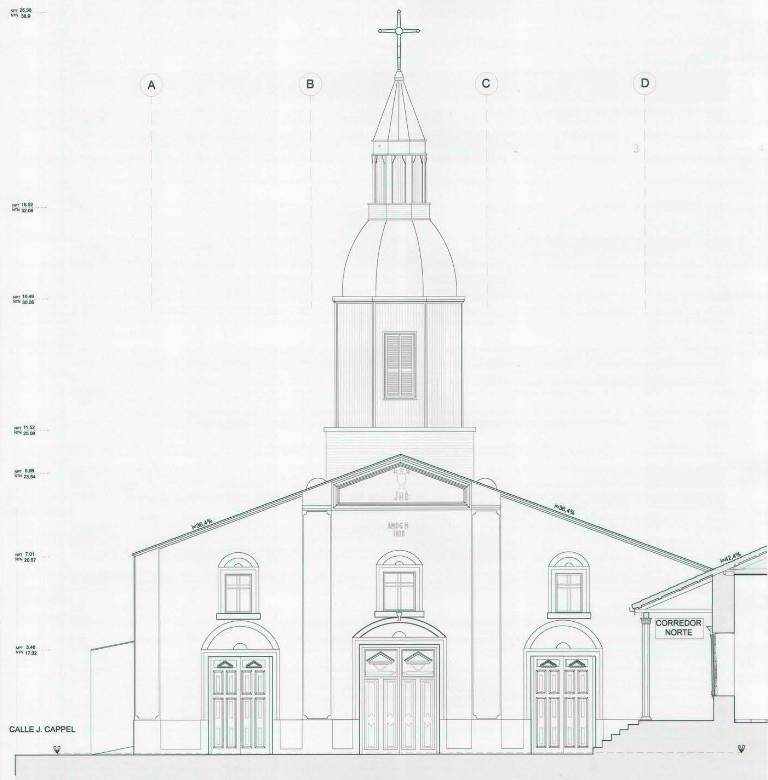
ELEVACIÓN PRINCIPAL [PONIENTE] ESC 1:75
