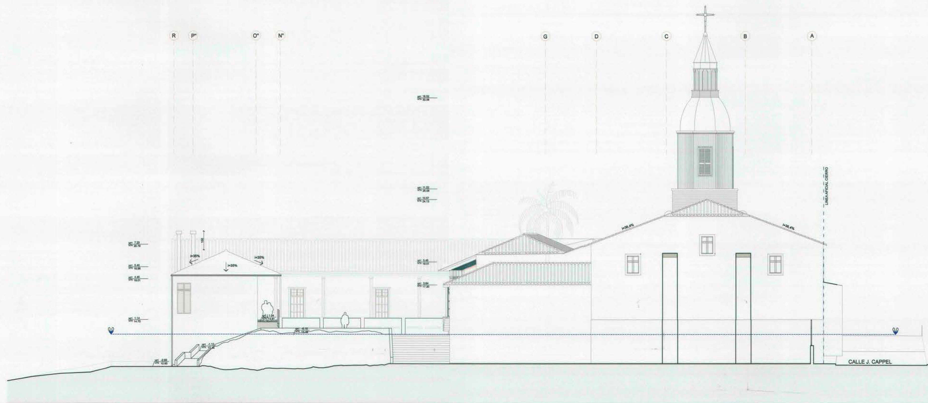
ELEVACIÓN OESTE ESC 1:150
