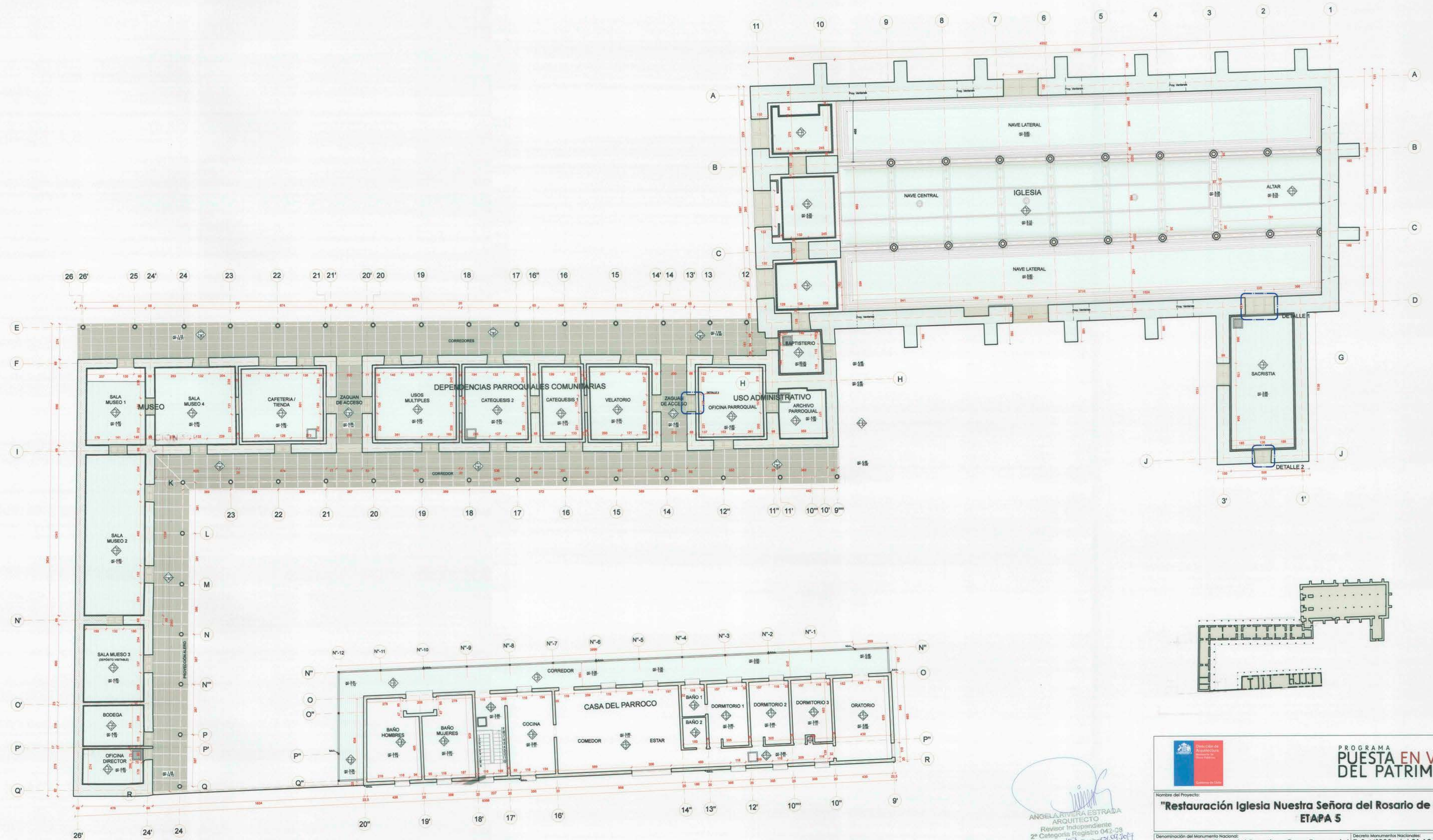
PLANTA GENERAL CIELOS ESC 1:150
