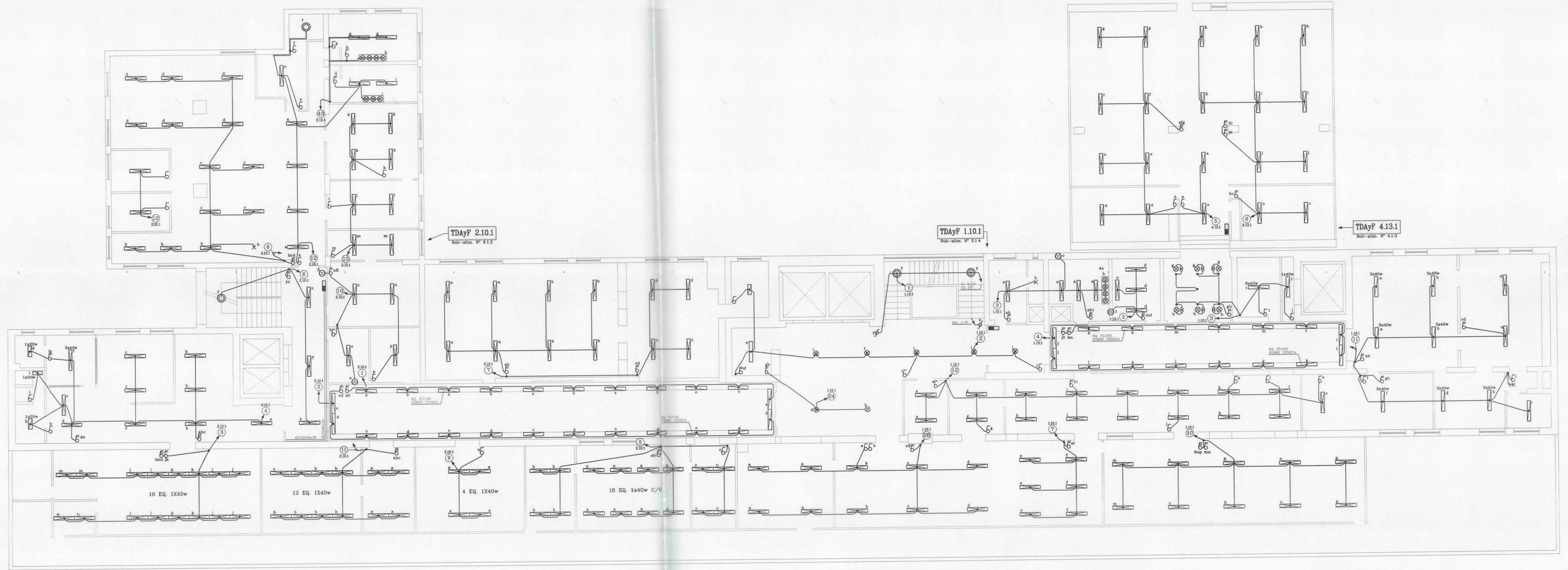
PLANTA ALUMBRADO DECIMO PISO ESCALA 1/100
