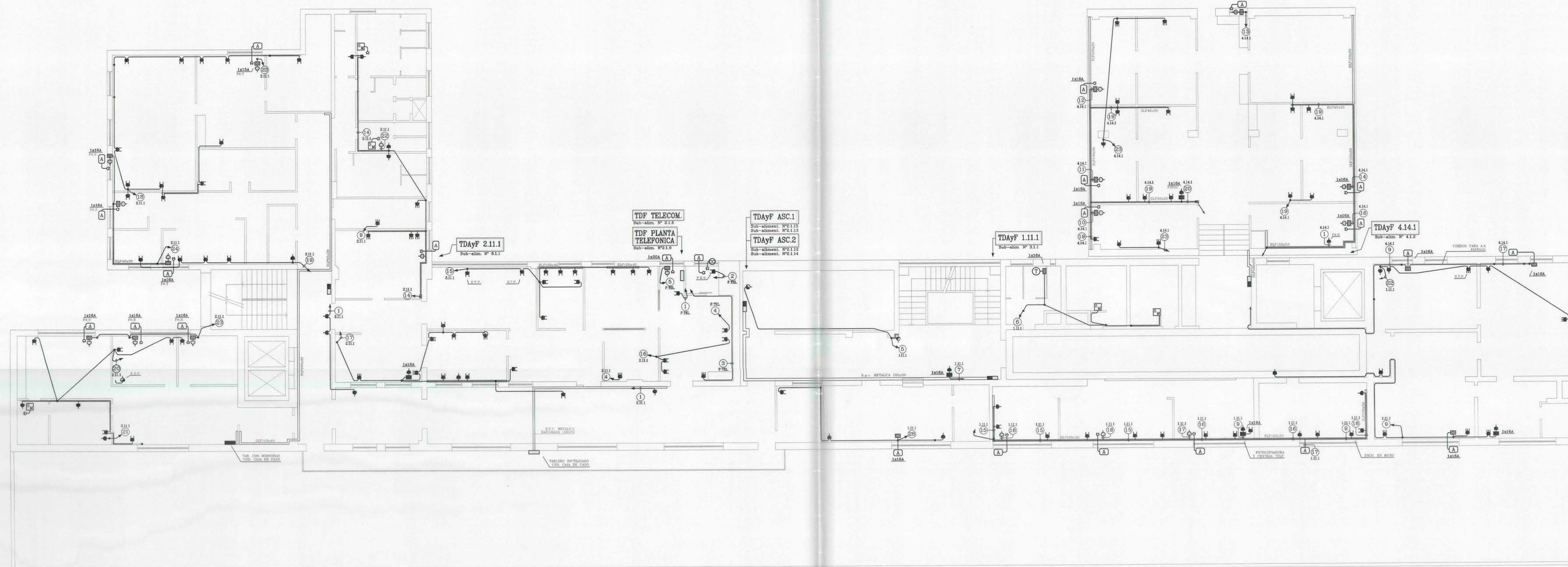
PLANTA ENCHUFES ONCEAVO PISO ESCALA 1/100
