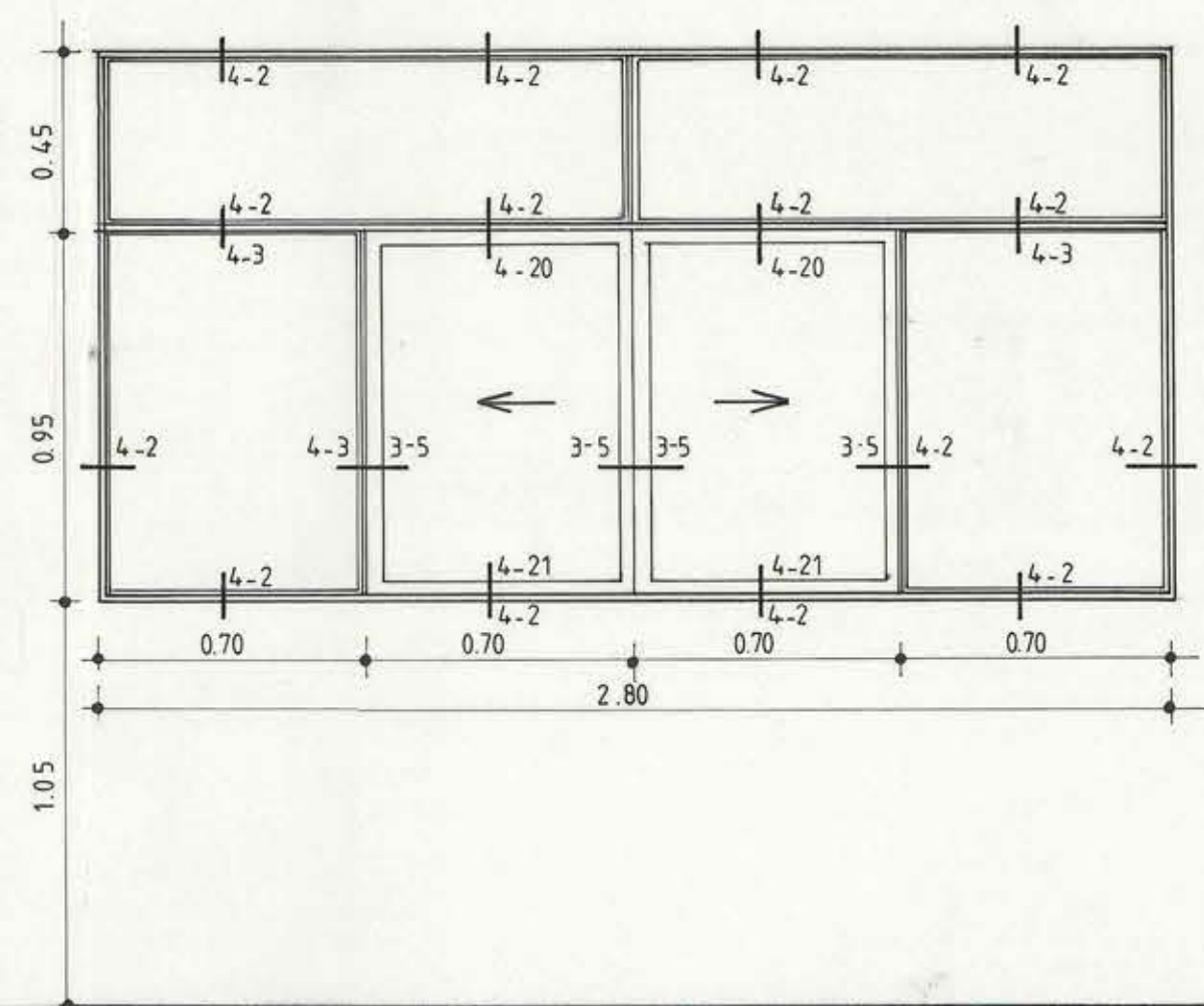
VENTANA V1 (SON 6) ESC. 1:20
