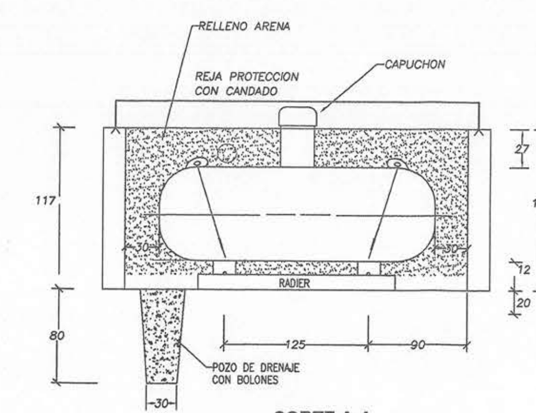
CORTE A-A
