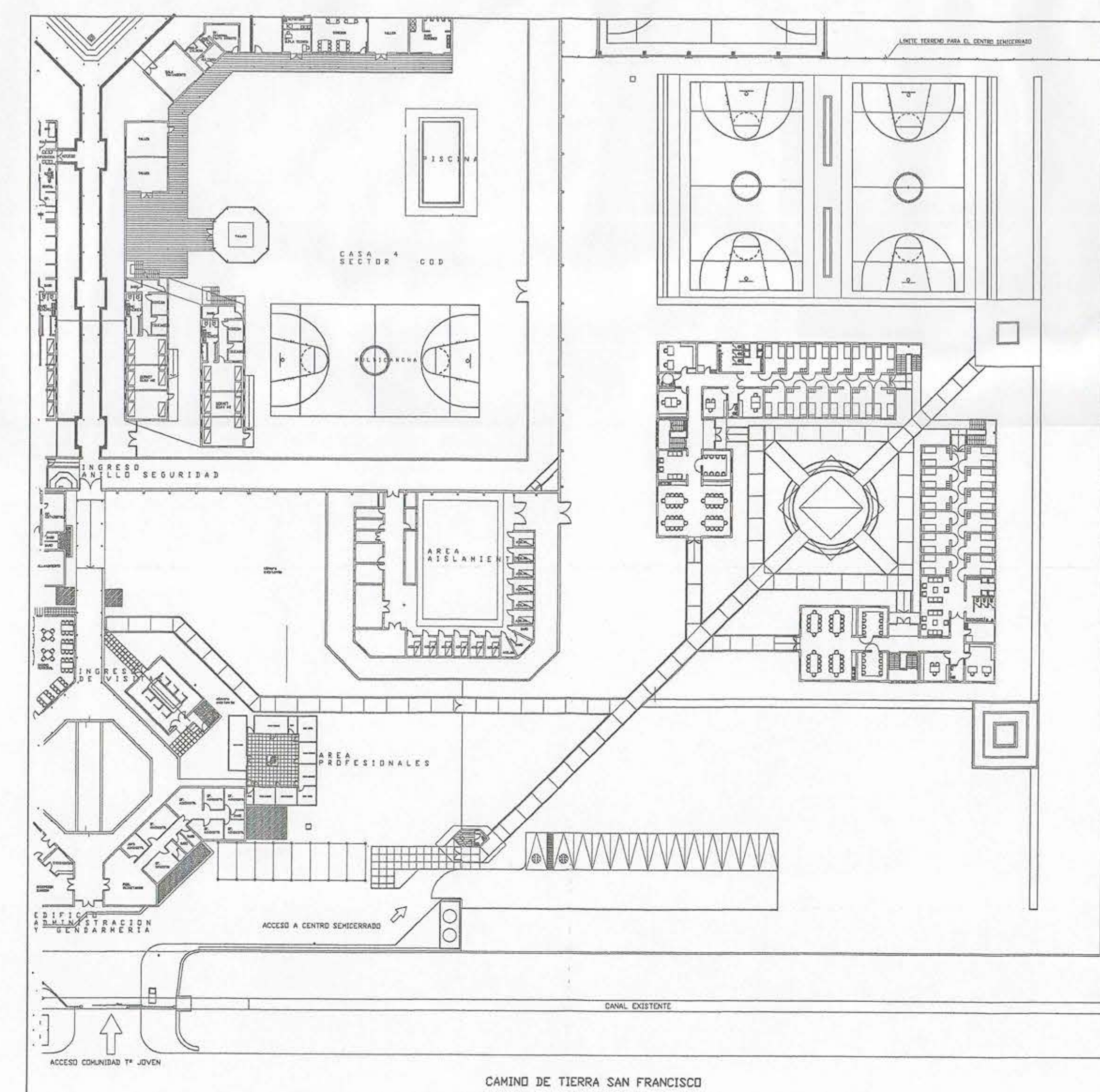
PLANTA EMPLAZAMIENTO ESC. 1:500
