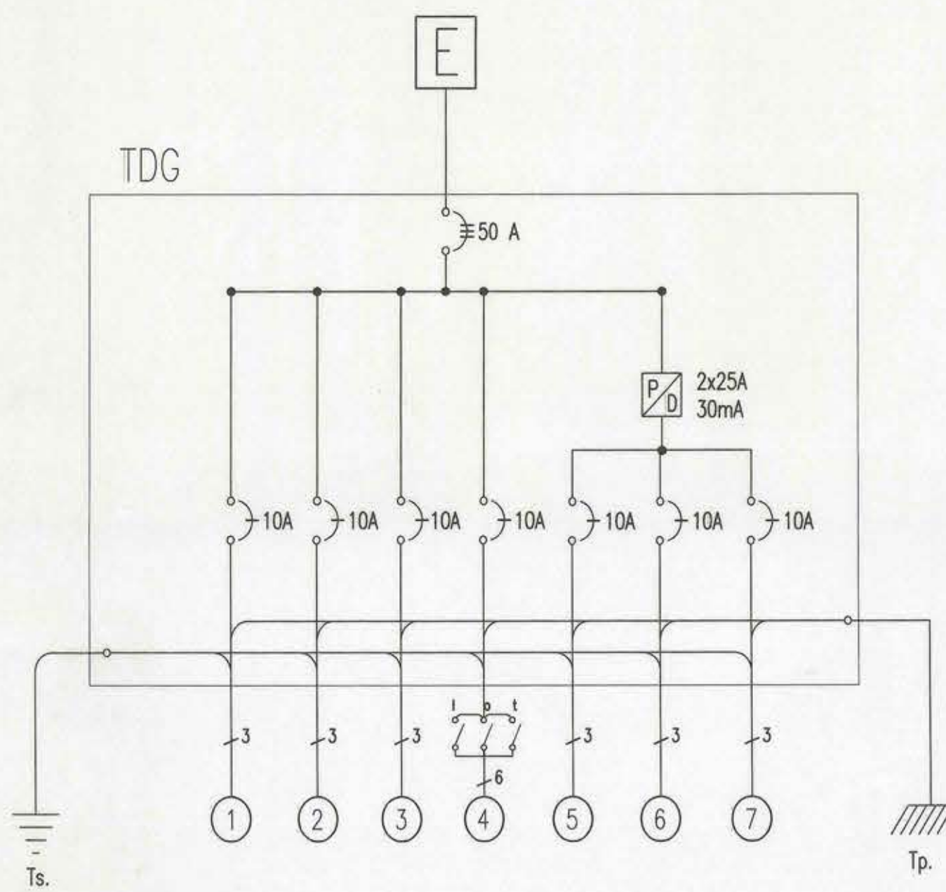
DIAGRAMA UNILINEAL TDG PARTE PROYECTADA
