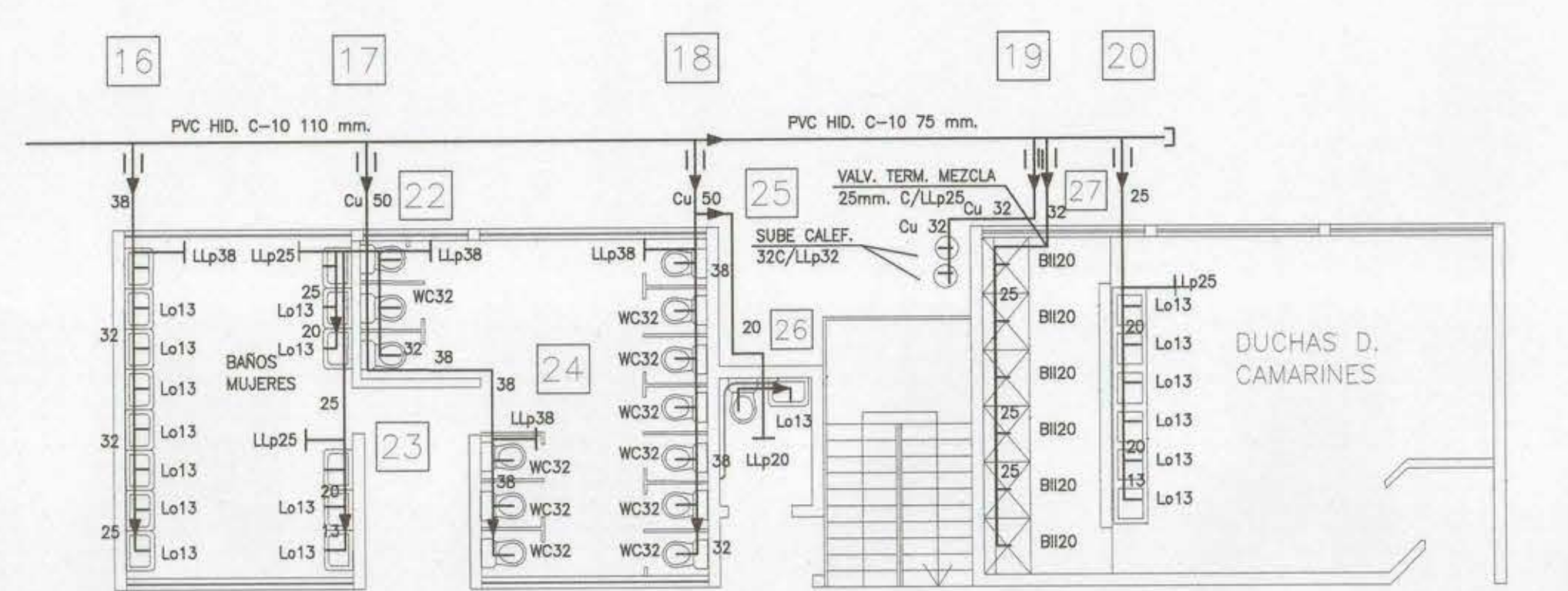
BAÑOS Y CAMARINES MUJERES ESCALA 1:100
