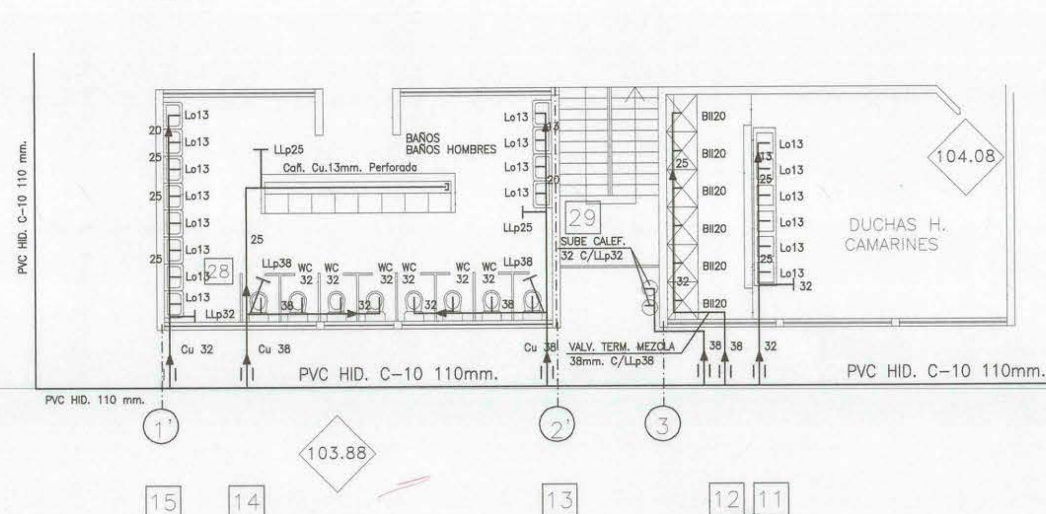
BAÑOS Y CAMARINES HOMBRES ESCALA 1:100
