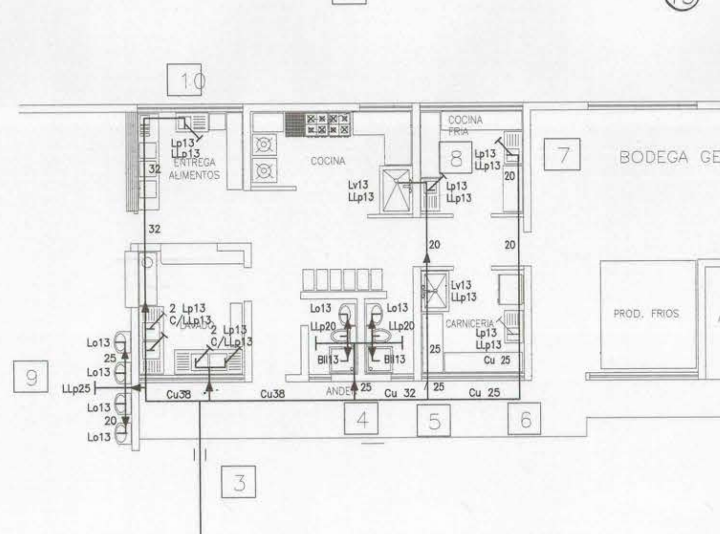
CASINO - COCINA ESCALA 1:100
