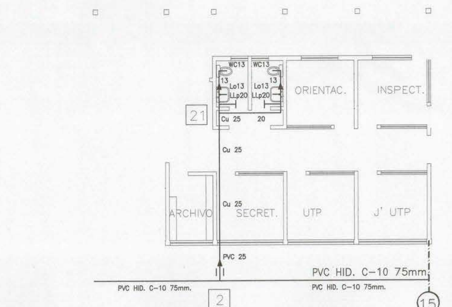
ADMINISTRACION ESCALA 1:100
