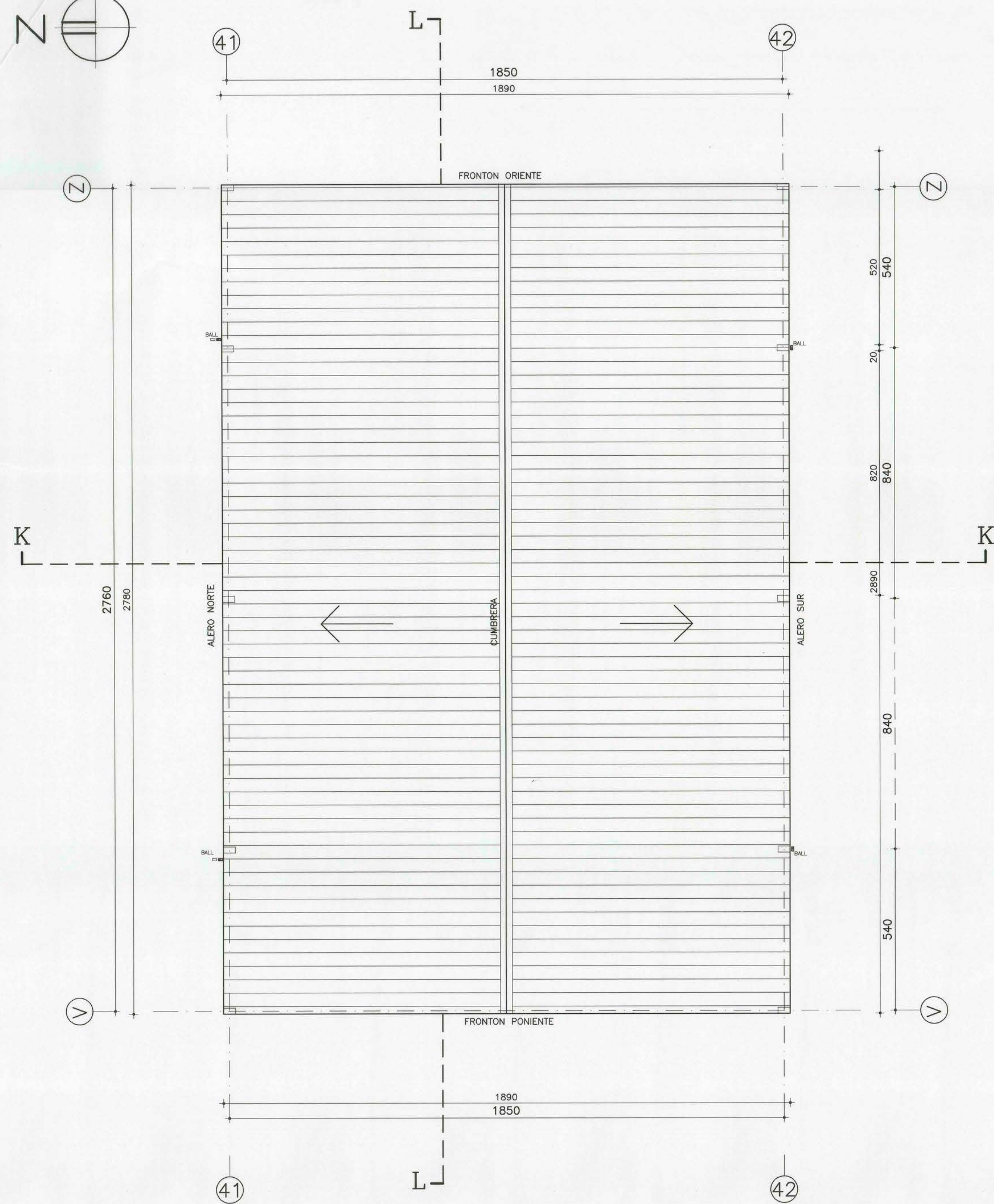
PLANTA CUBIERTA ESCALA 1/75
