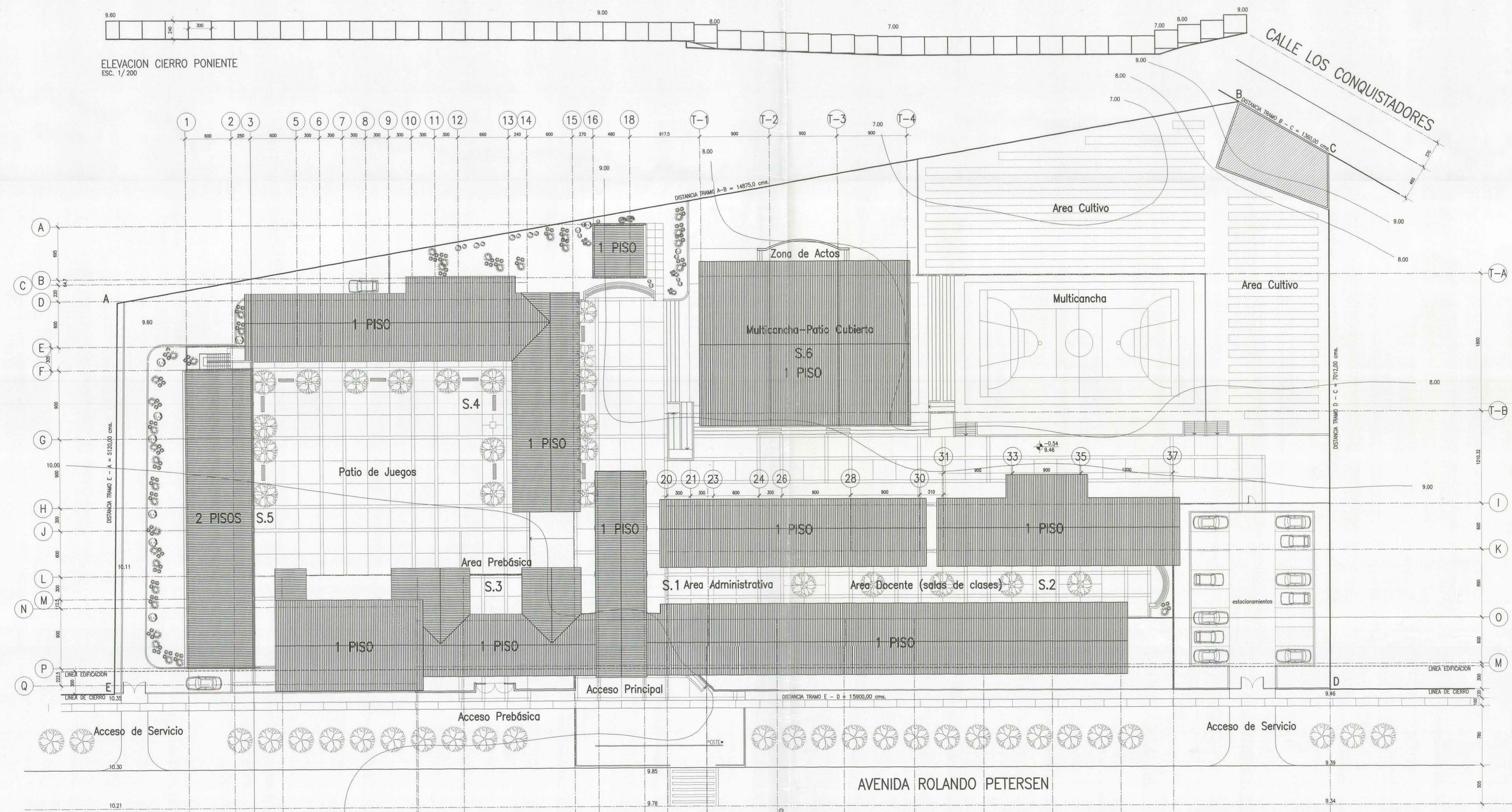
PLANTA GENERAL DE TECHUMBRE ESC. 1/200
