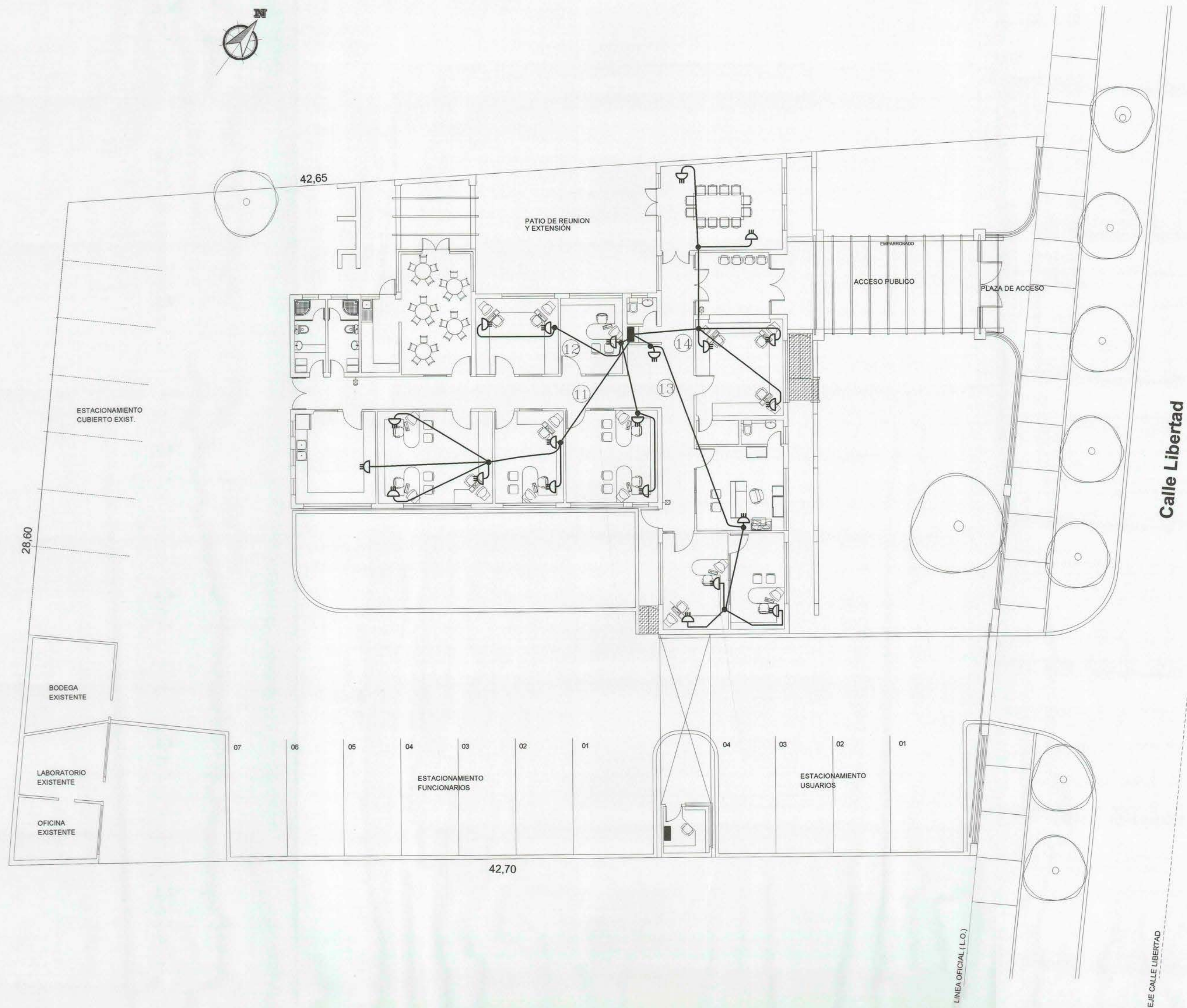
PLANTA GENERAL DE ENCHUFES DE COMPUTACION ESCALA 1/100
