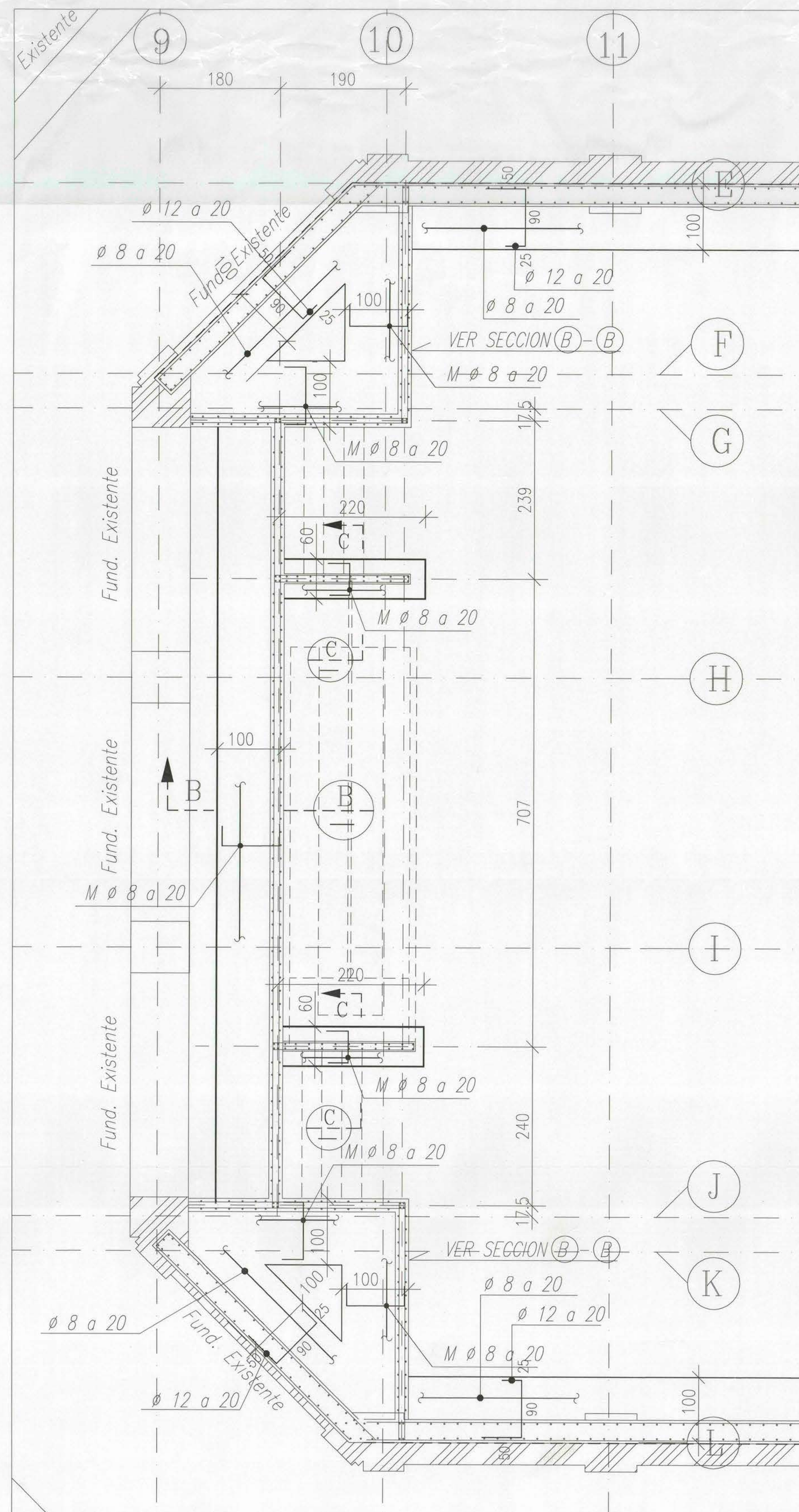
PLANTA DE FUNDACIONES MUROS DE CONTENCION SECTOR RAMPA (ZOCALO N-4.90)
