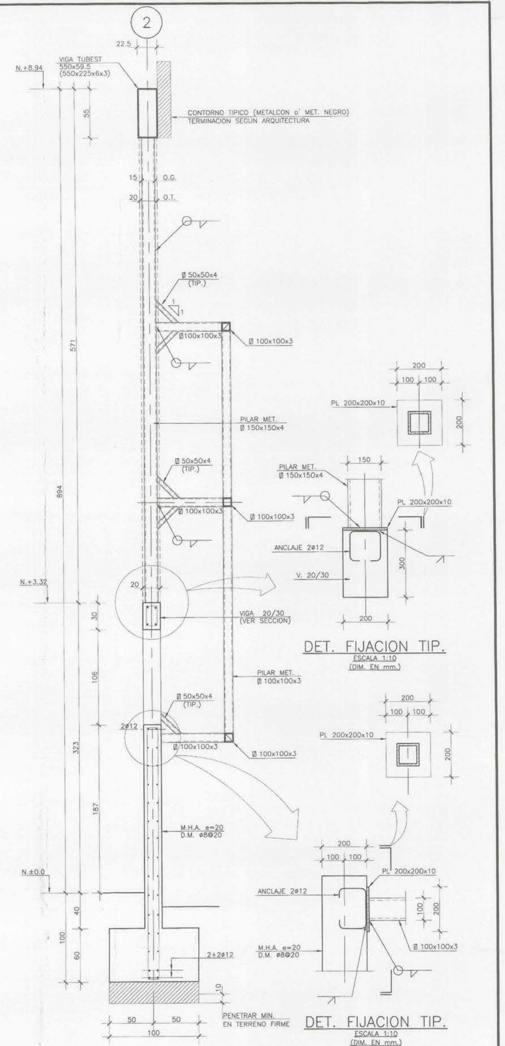
(ESCAZILLON OBRA GRUESA) SECCION B - B ESCALA 1:25
