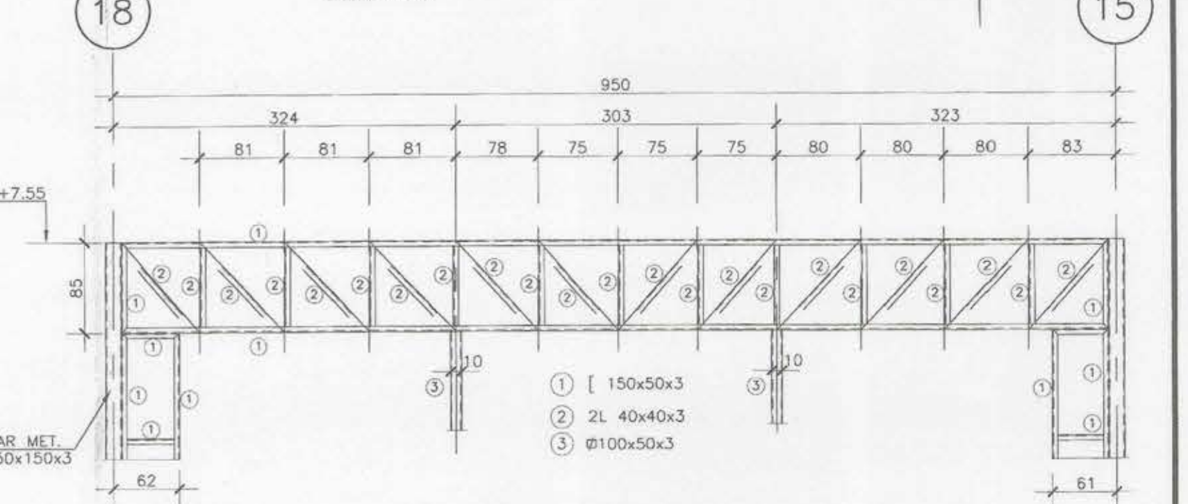
(ENTRE 18 Y 15) ELEVACION VIGA ENREJADA 15/85 EJE A ESCALA 1:50
