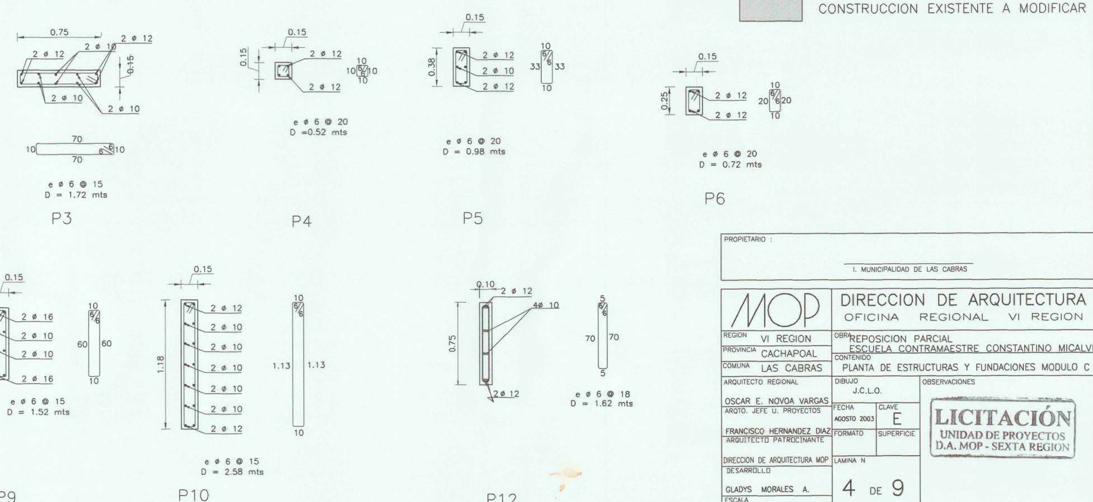
PLANTA DE ESTRUCTURAS MODULO C ESCALA 1 : 50
