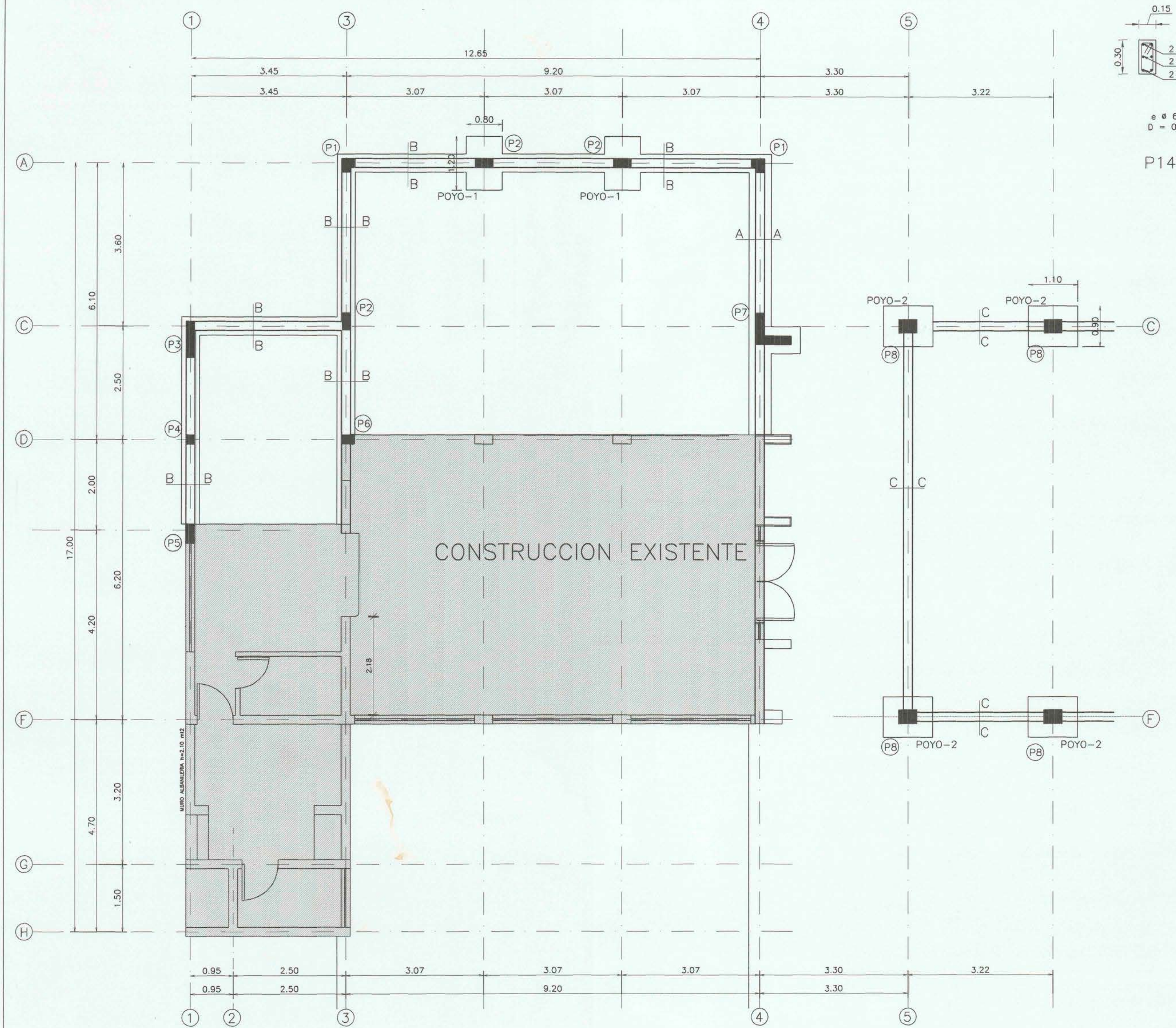
PLANTA DE FUNDACIONES MODULO C ESCALA 1 : 50
