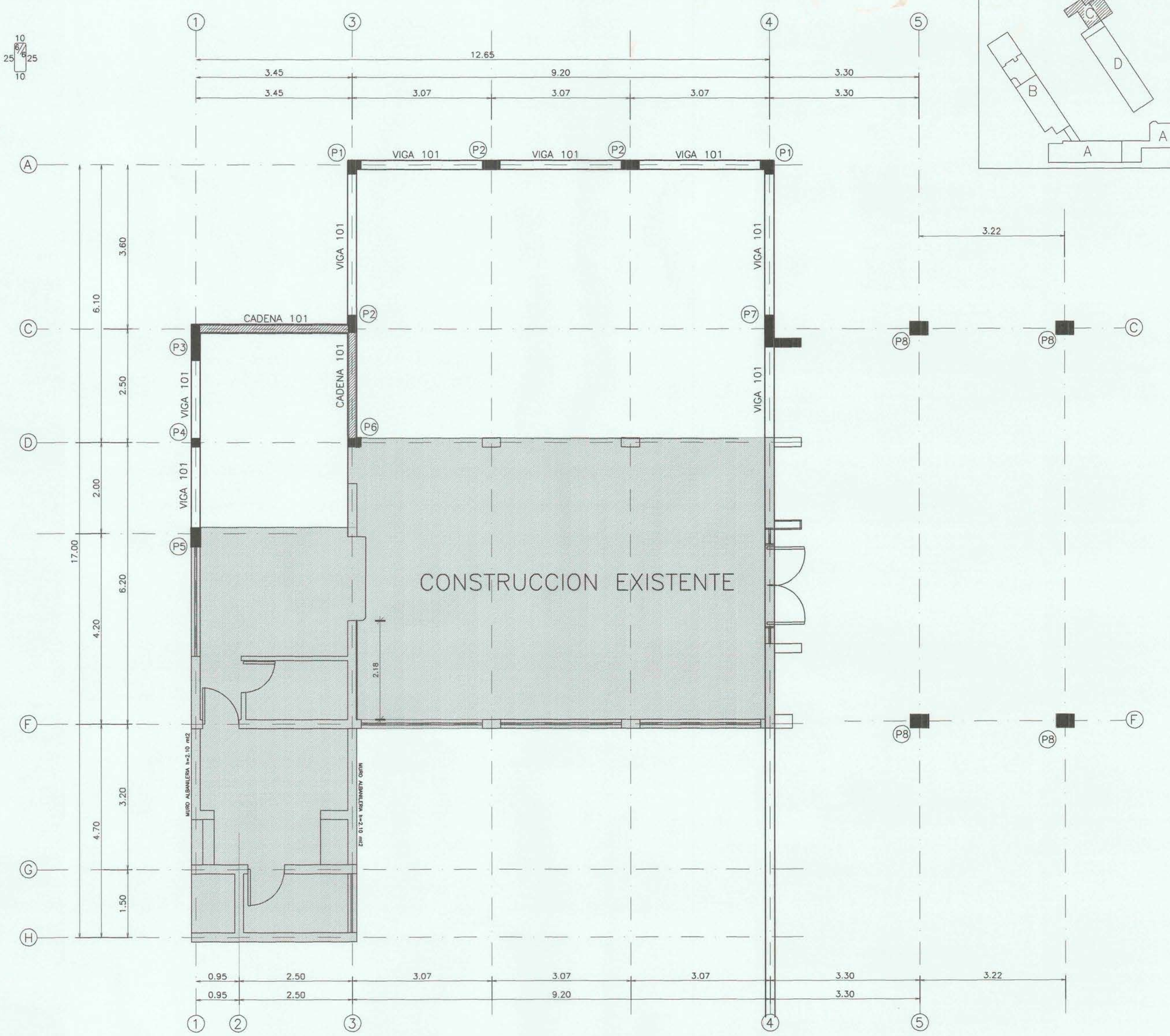
PLANTA DE ESTRUCTURAS MODULO C ESCALA 1 : 50
