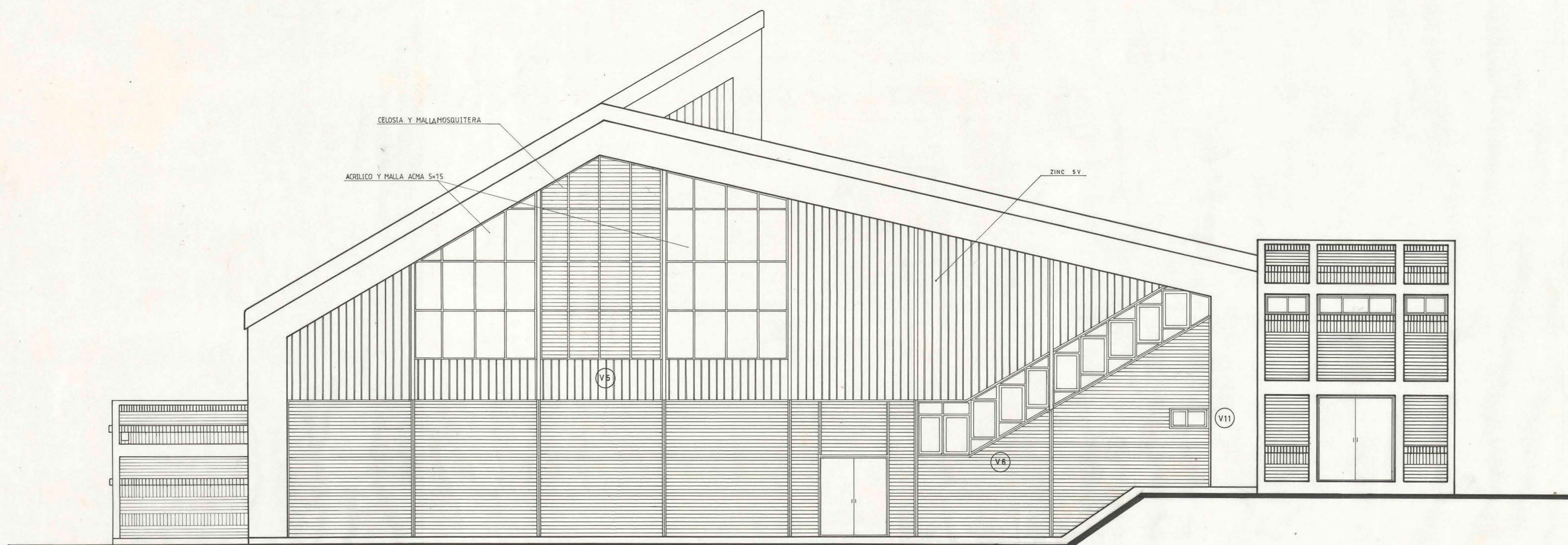
ELEVACION SUR ESCALA 1/50
