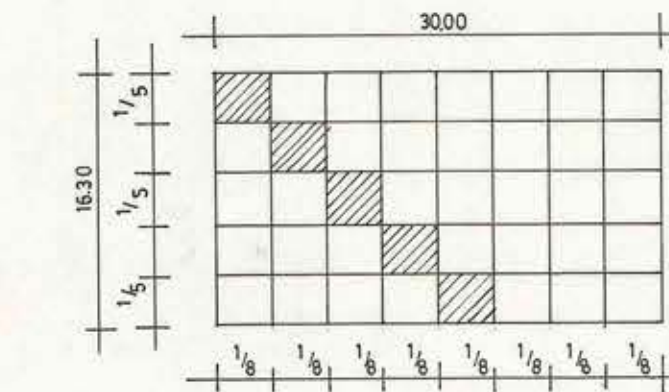
DET. HORMIGONADO DE CANCHA POR PAÑOS ALTERNADOS ESCALA 1/500
