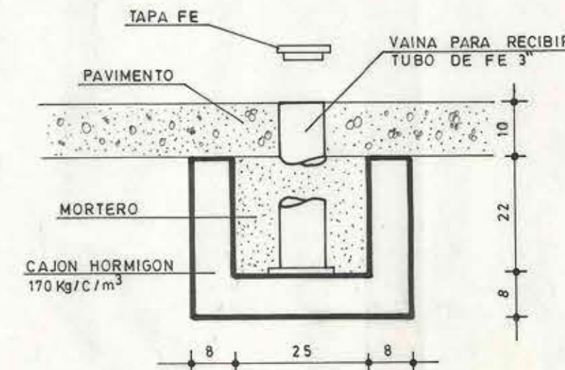
DET. EMPOTRAMIENTO TUBO PARA VOLEIBOL ESCALA 1/10
