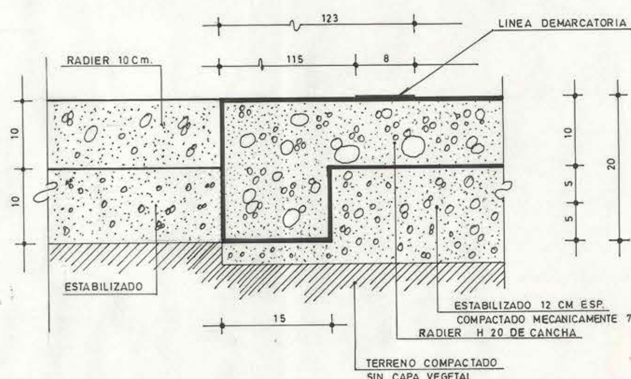
CORTE A-A ESCALA 1/5
