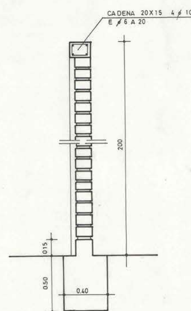
CORTE Z-Z ESCALA 1/20
