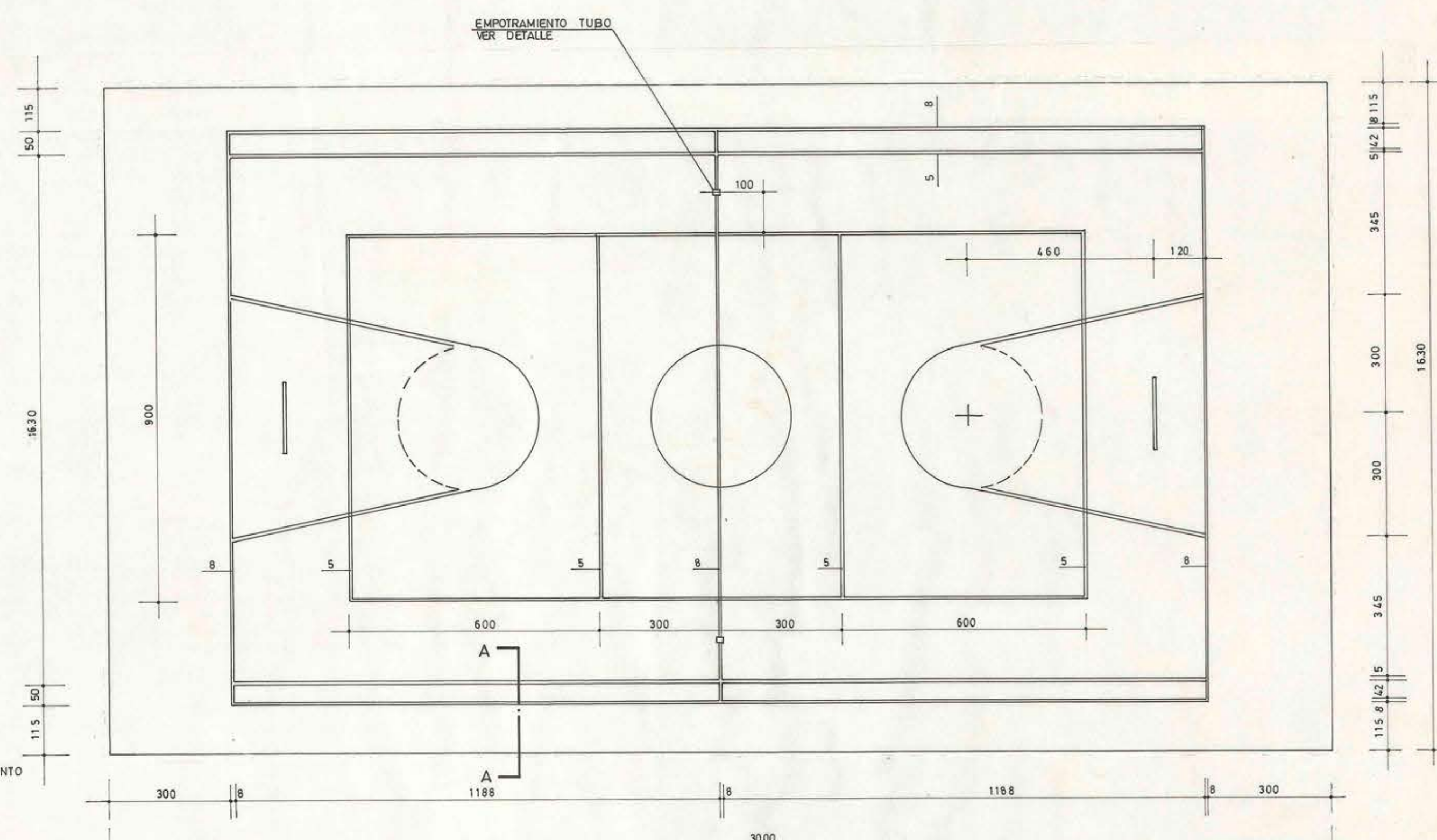
PLANTA MULTICANCHA ESCALA 1/100
