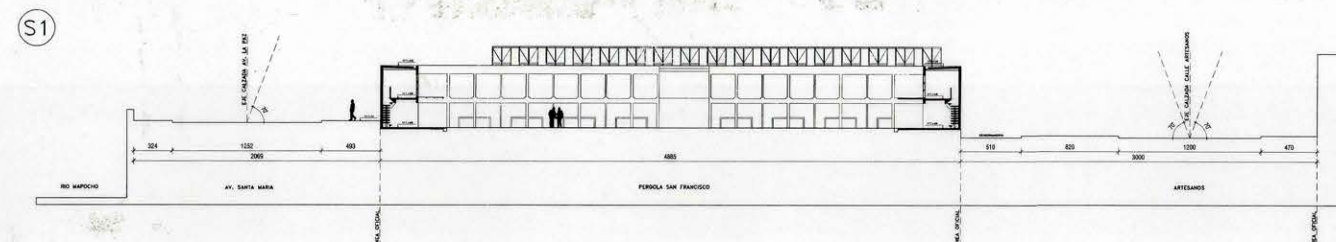
SILUETA CORTE PONIENTE PERGOLA SAN FRANCISCO 1:200
