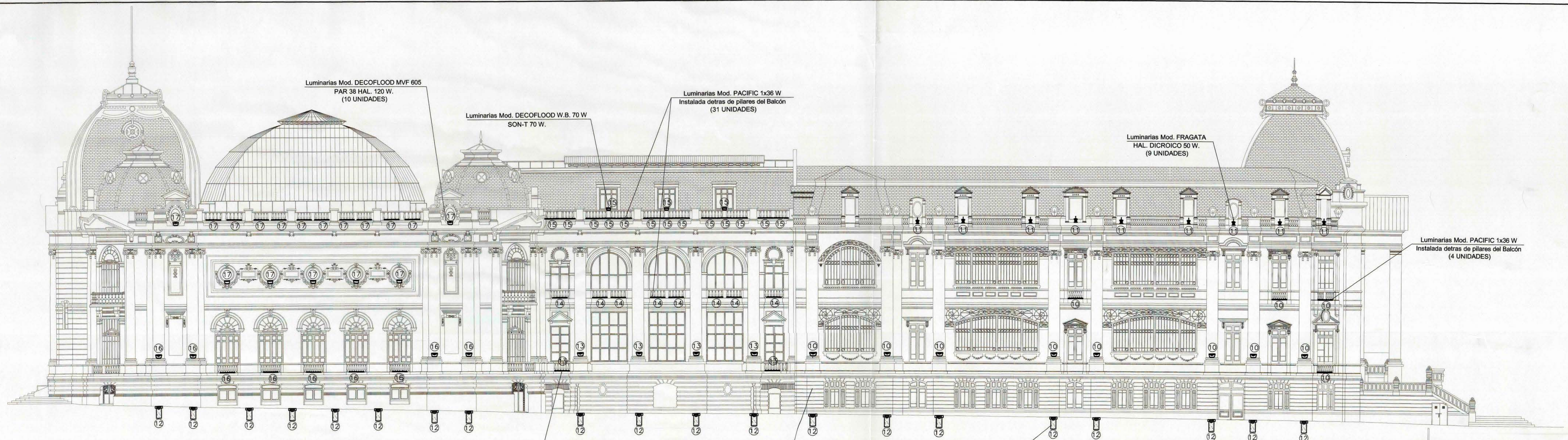
FACHADA NORTE Esc. 1:125
