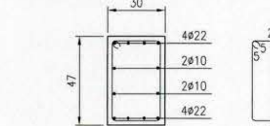
DETALLE PILAR P107 ESC. 1:20
