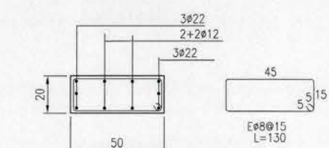
DETALLE PILAR P104 ESC. 1:20
