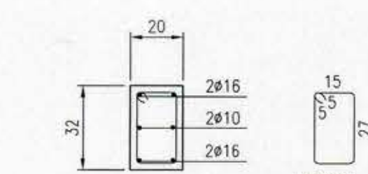
DETALLE VIGA V101 ESC. 1:20
