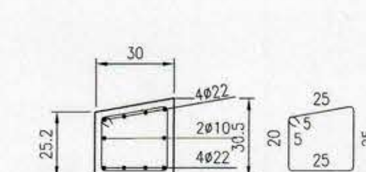
DETALLE PILAR P105 ESC. 1:20
