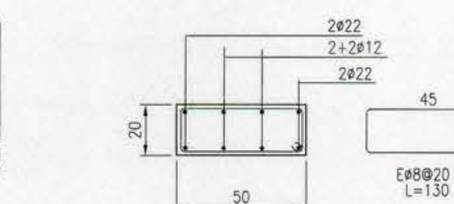
DETALLE PILAR P004 ESC. 1:20
