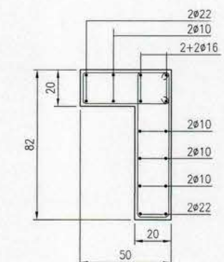
DETALLE PILAR P103 ESC. 1:20
