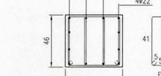
DETALLE PILAR P002 ESC. 1:20
