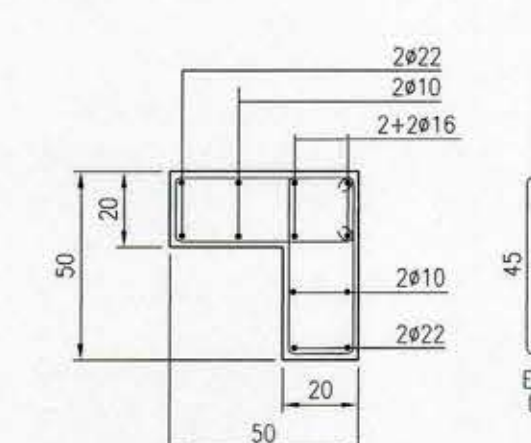
DETALLE PILAR P102 ESC. 1:20
