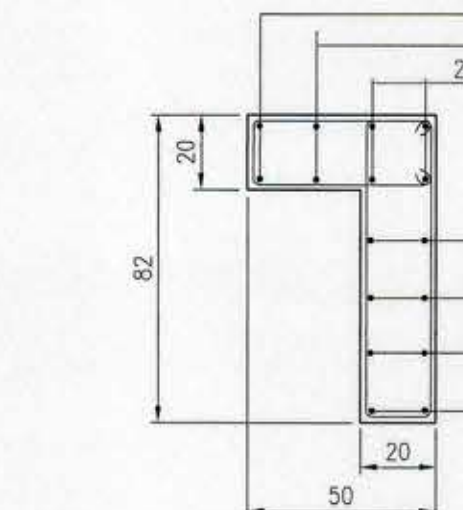
DETALLE PILAR P003 ESC. 1:20
