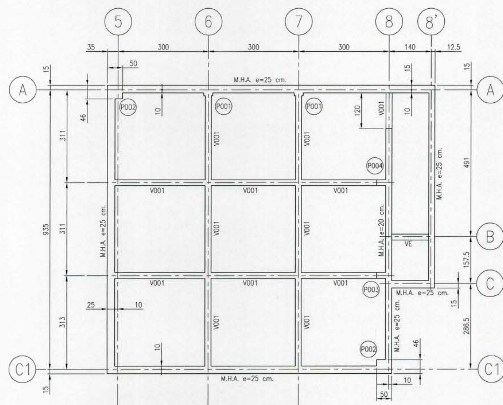
PLANTA DE ESTRUCTURA SUBTERRANEO ESC. 1:75
