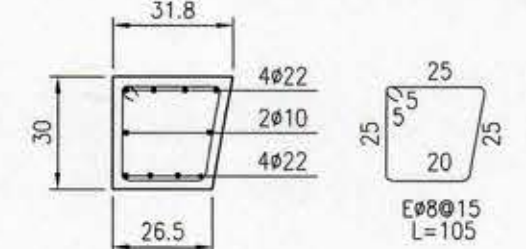
DETALLE PILAR P106 ESC. 1:20
