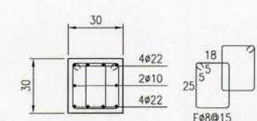
DETALLE PILAR P001 ESC. 1:20
