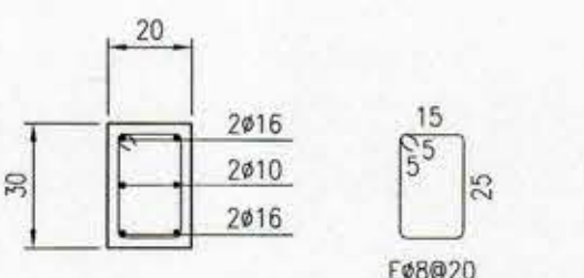
DETALLE VIGA V001 ESC. 1:20
