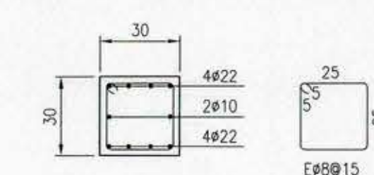
DETALLE PILAR P101 ESC. 1:20
