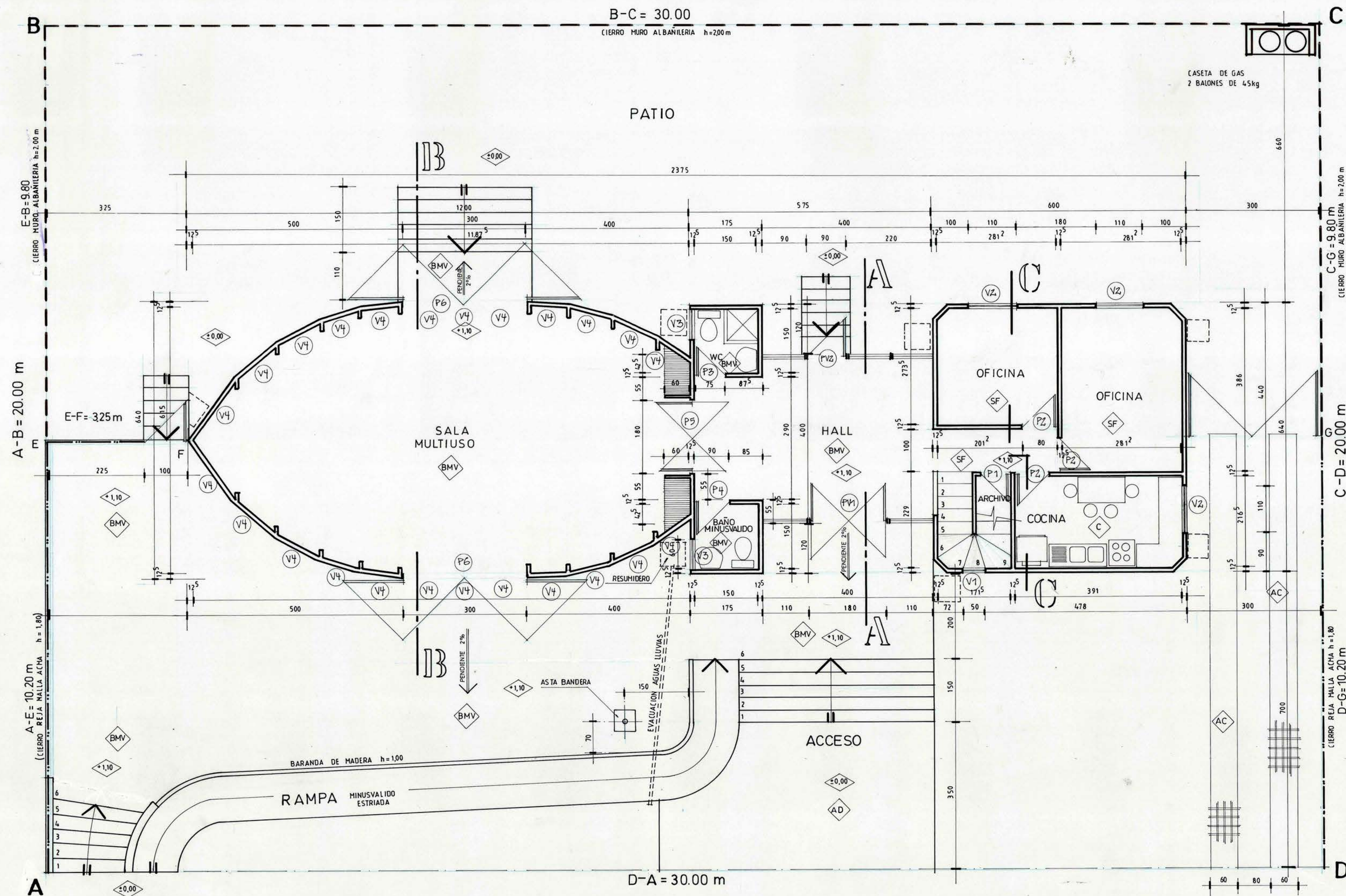
PLANTA ARQUITECTURA 1º PISO ESCALA 1/50 EMPLAZAMIENTO
