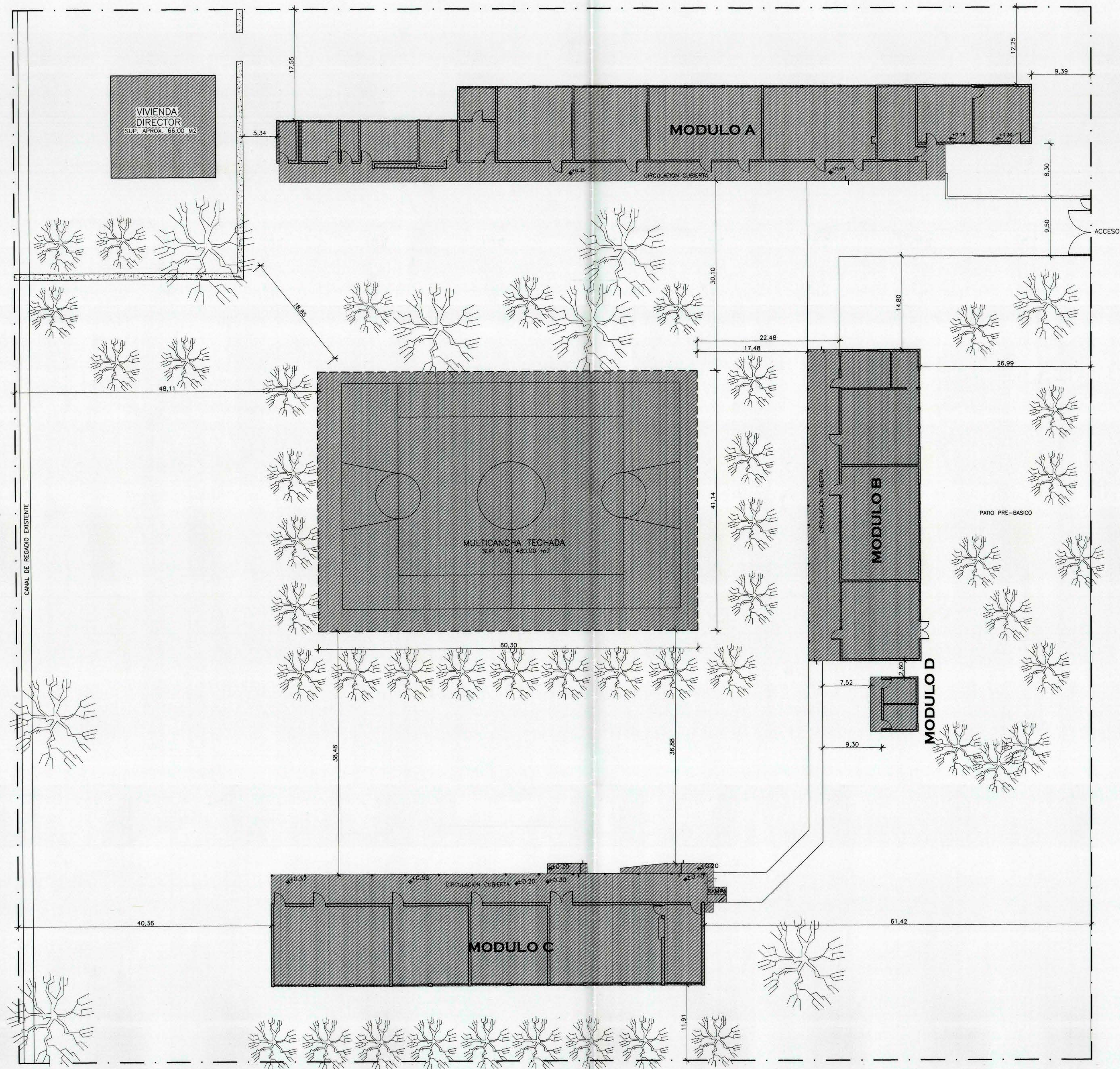
EMPLAZAMIENTO GENERAL ESCALA 1:125
