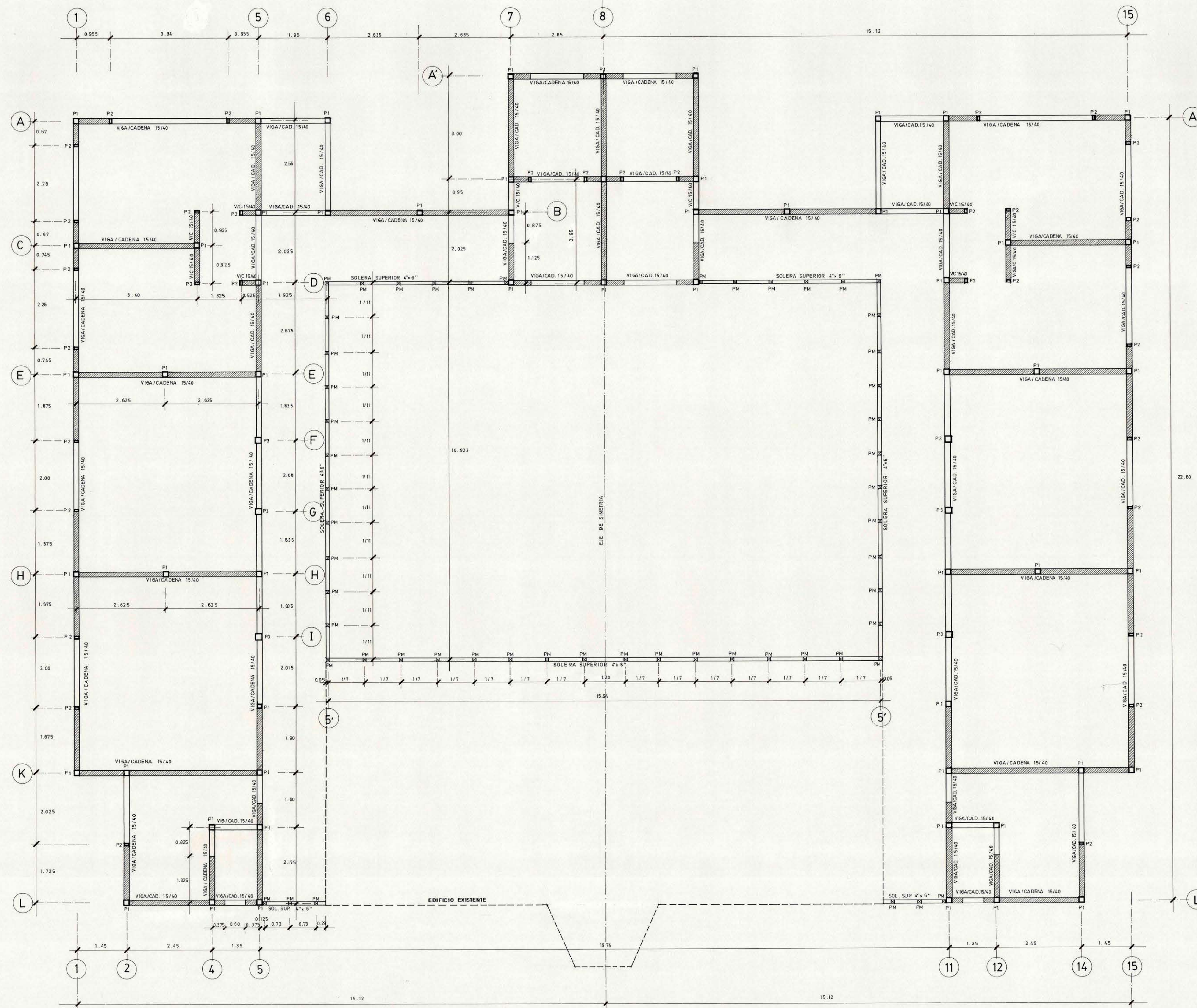
PLANTA DE ESTRUCTURAS
