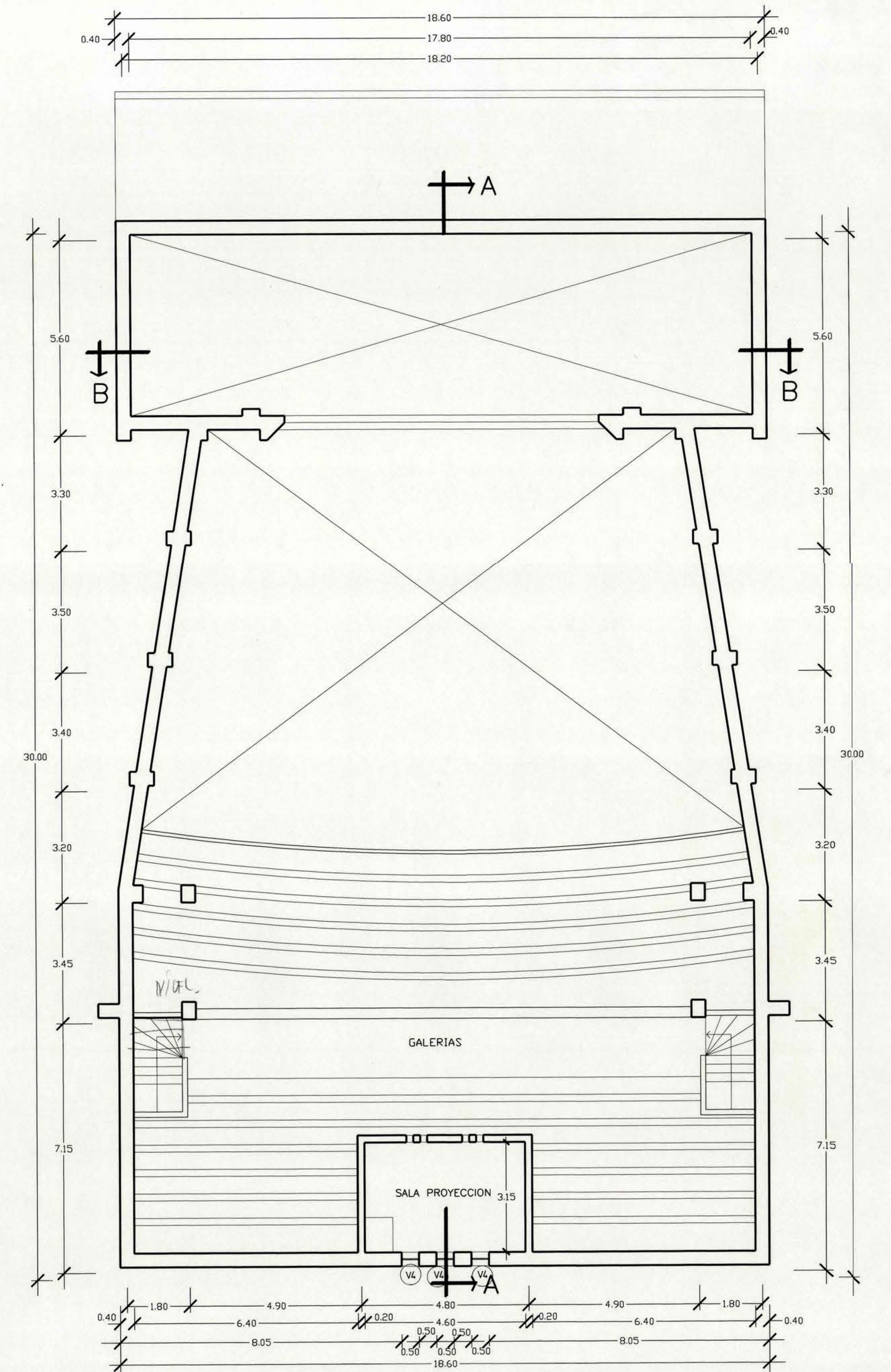
PLANTA ARQUITECTURA 3er PISO
