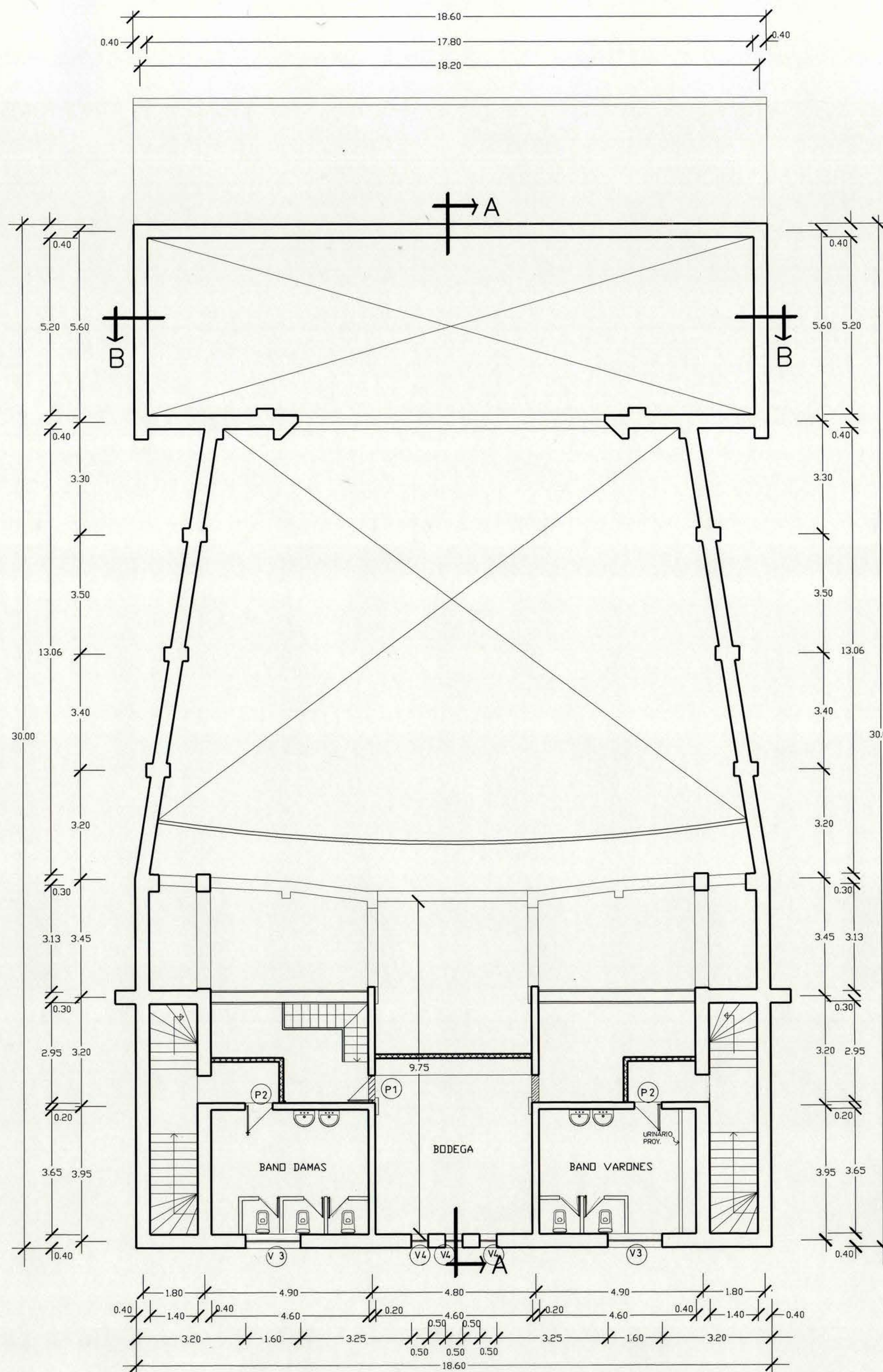
PLANTA ARQUITECTURA 2do PISO
