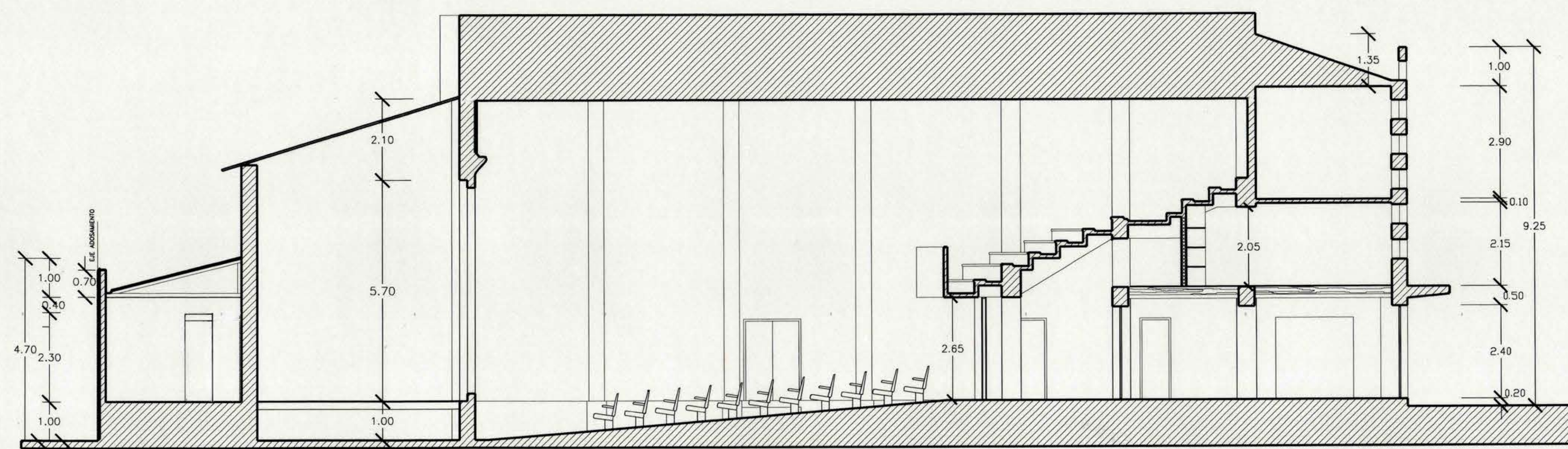
CORTE A - A
