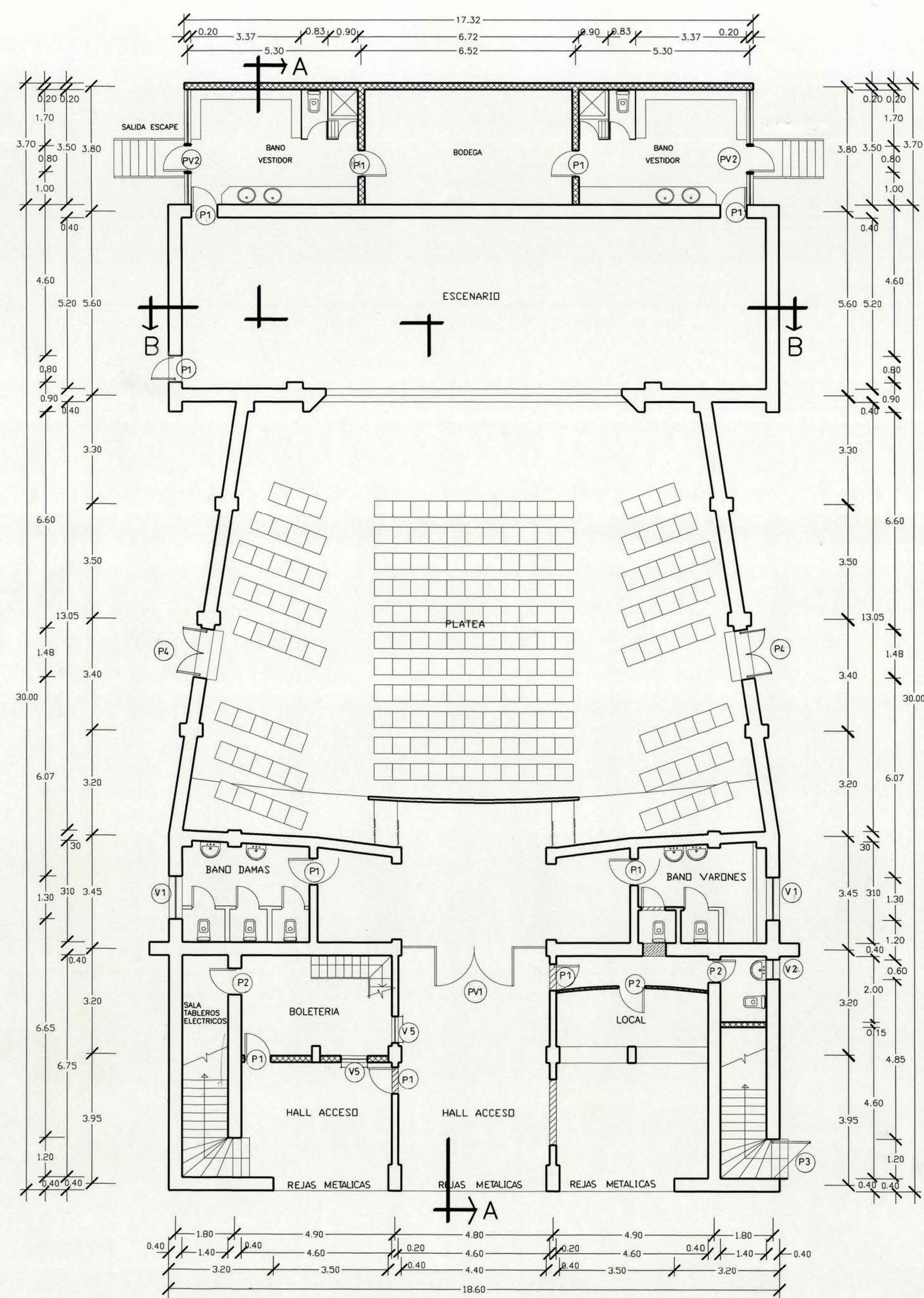
PLANTA ARQUITECTURA 1er PISO
