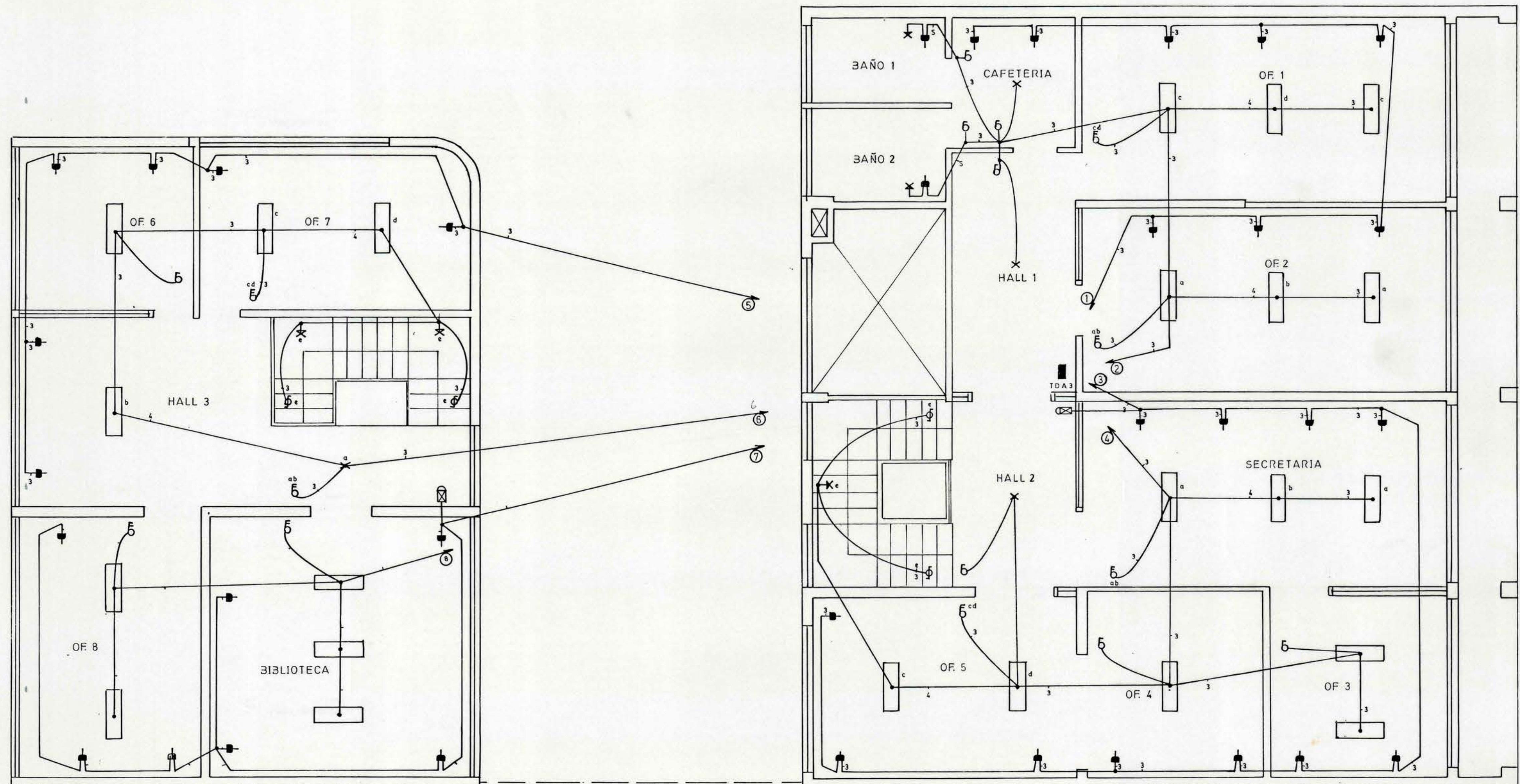
Sgdo. PISO
