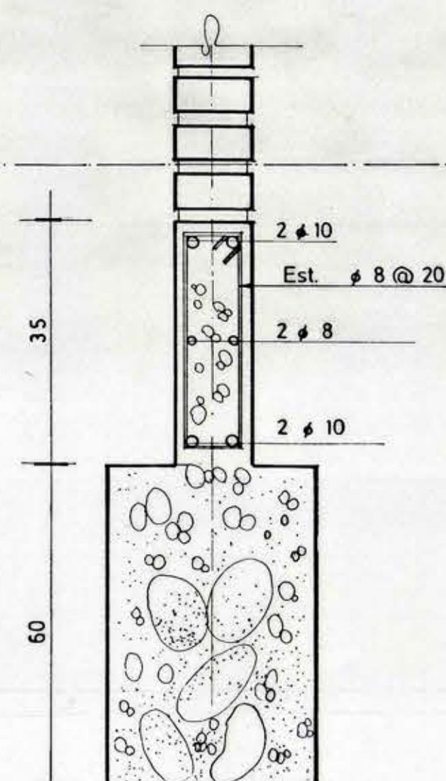
Corte D - D
