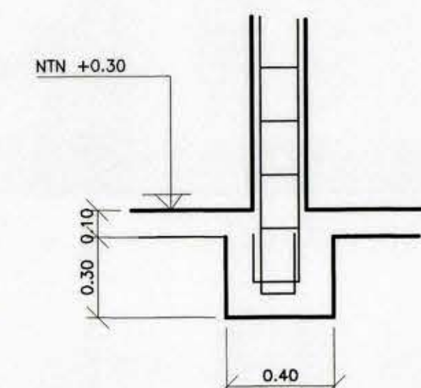
CORTE D-D ESCALA 1:20
