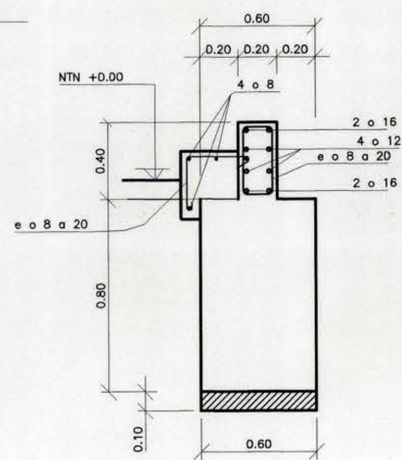
CORTE C-C ESCALA 1:20
