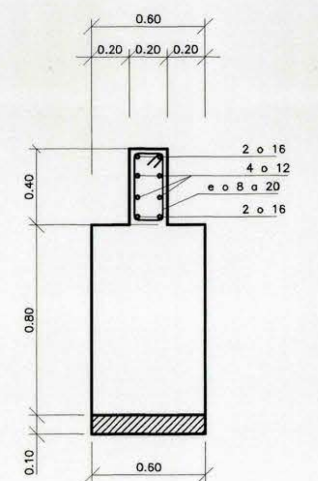
CORTE B-B ESCALA 1:20
