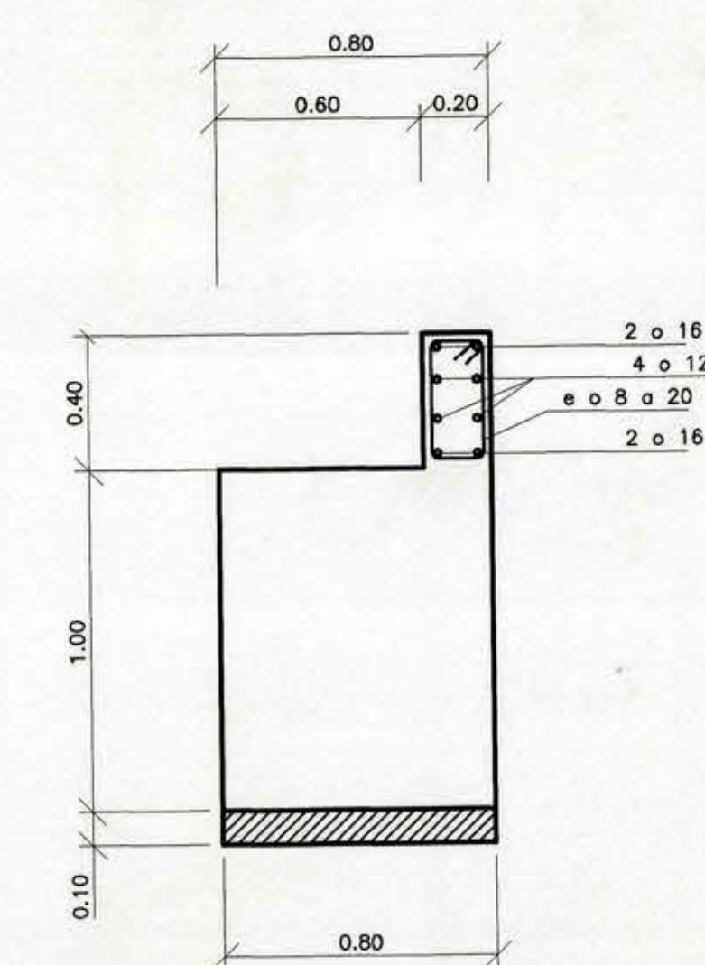
CORTE E-E ESCALA 1:20
