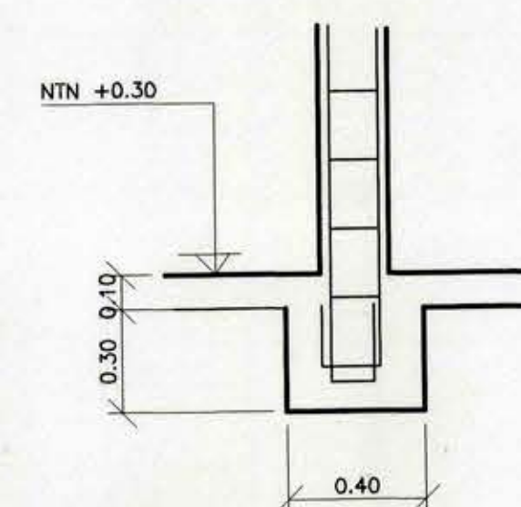
CORTE D-D ESCALA 1:20 (FUNDACIÓN POLIESTÓN)
