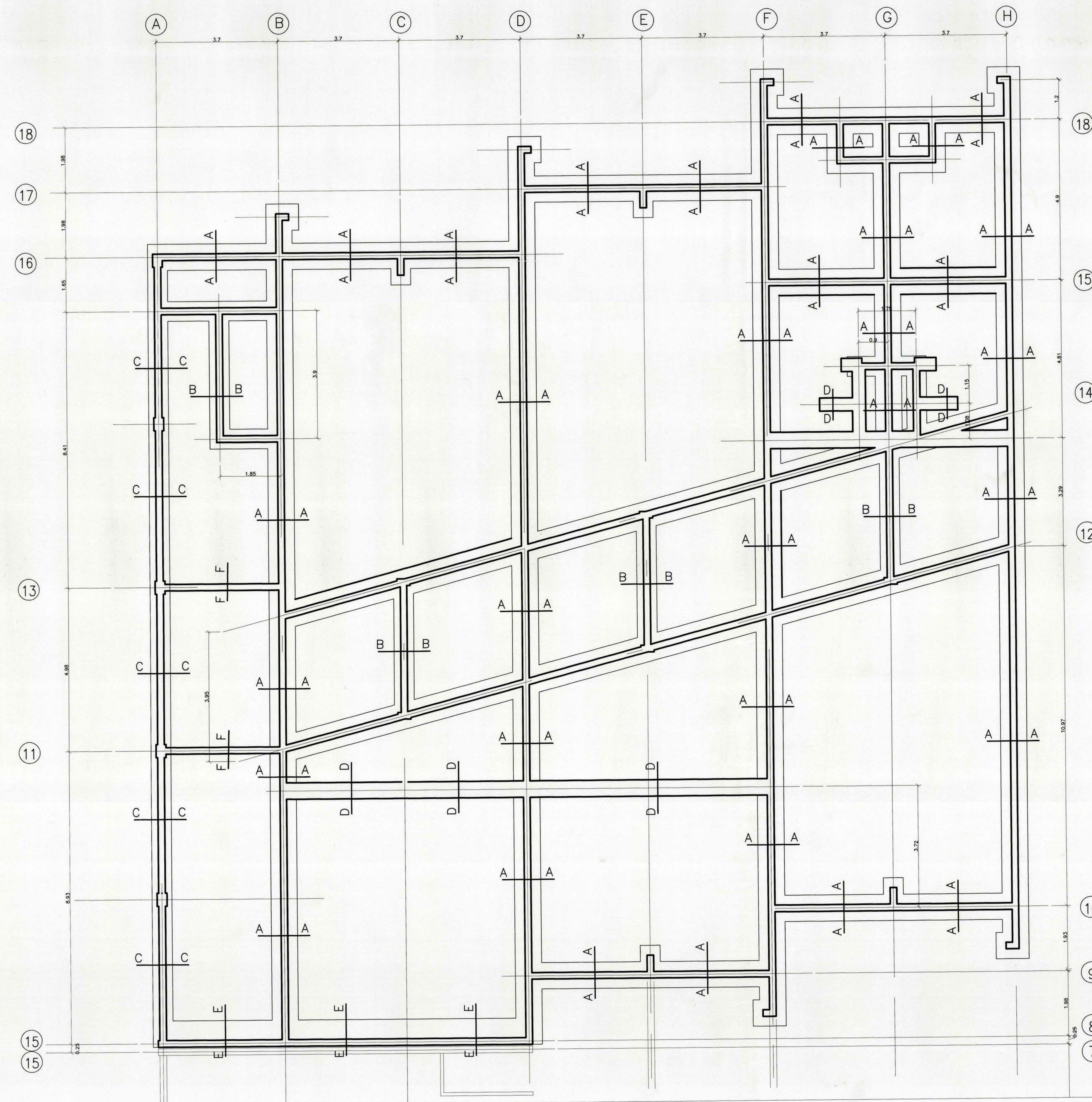
PLANTA FUNDACIONES MODULO A ESCALA 1 : 50
