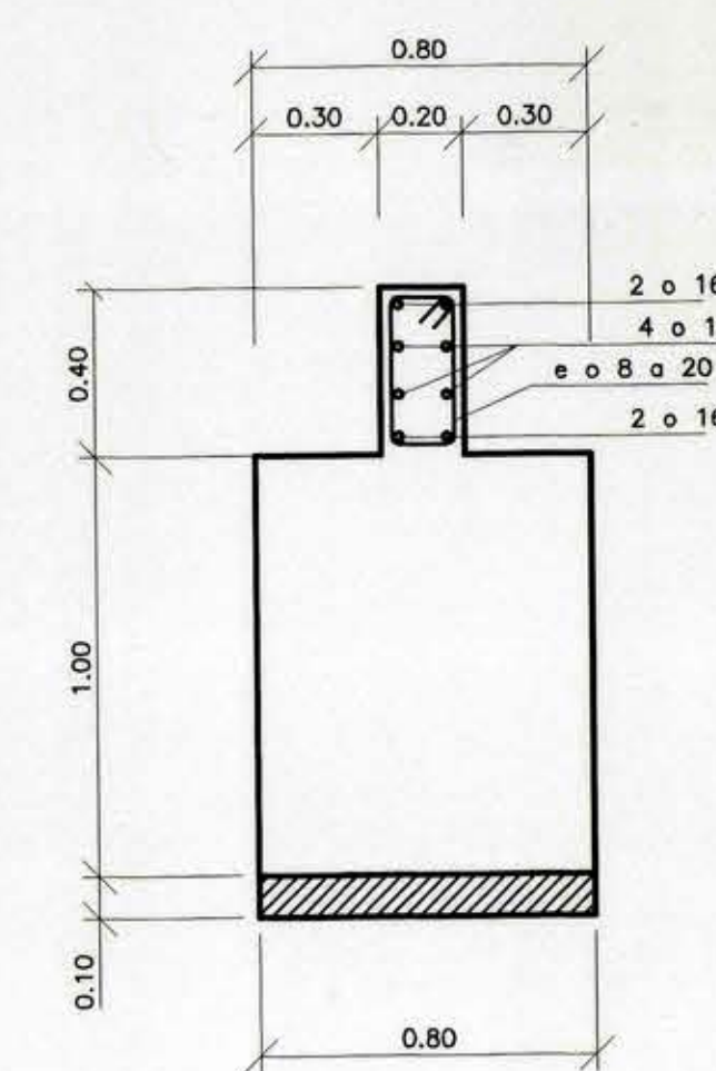
CORTE A-A ESCALA 1:20
