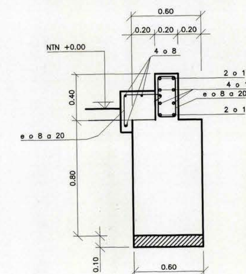
CORTE C-C ESCALA 1:20
