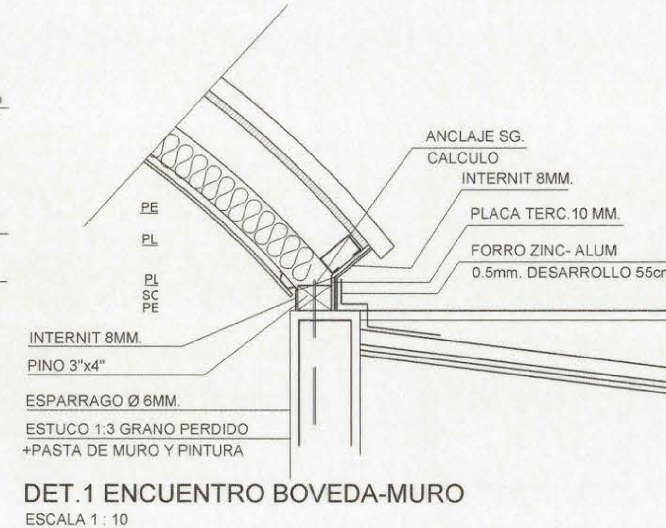
ESCANTILLON VIVIENDA
