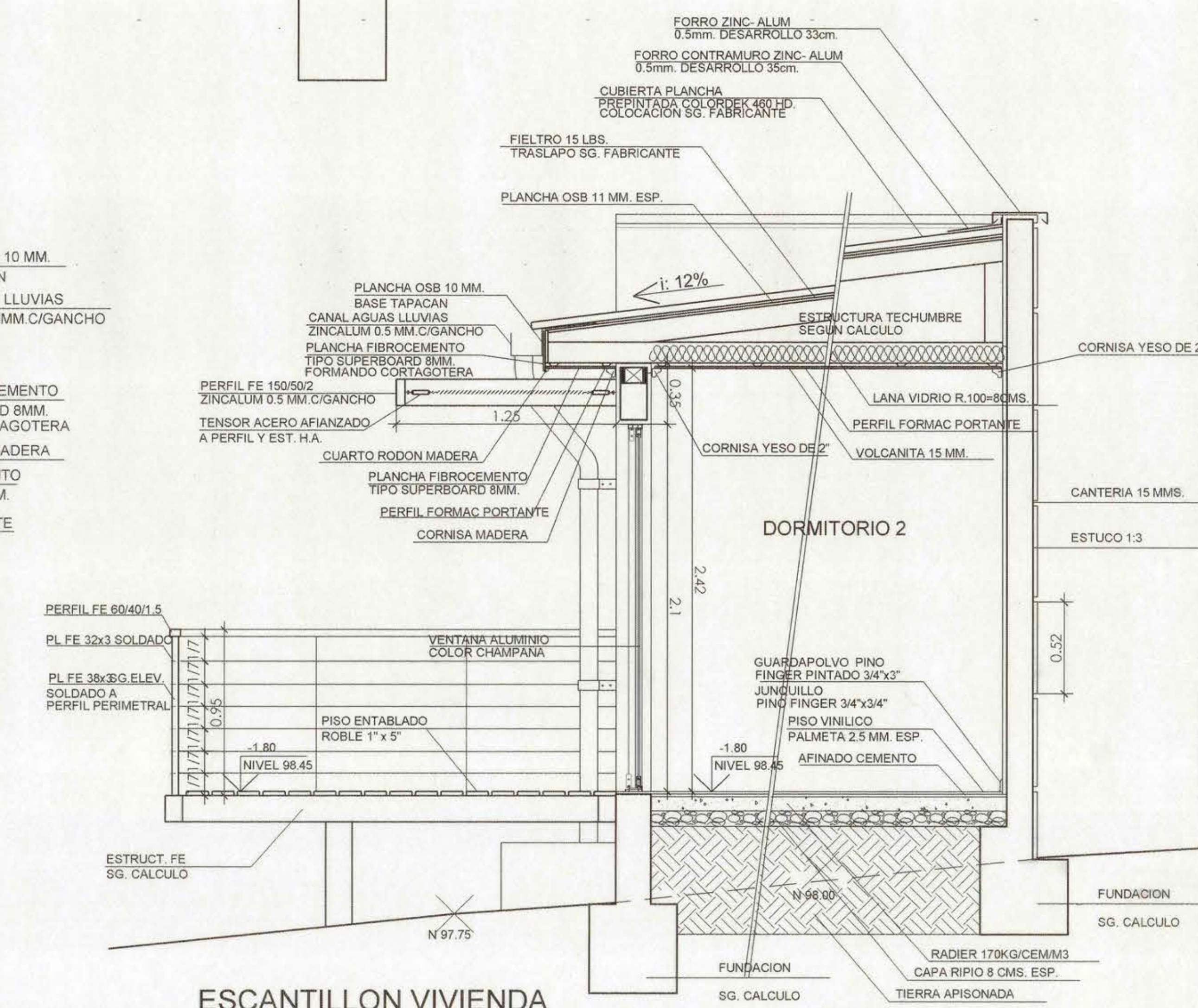
ESCANTILLON VIVIENDA
