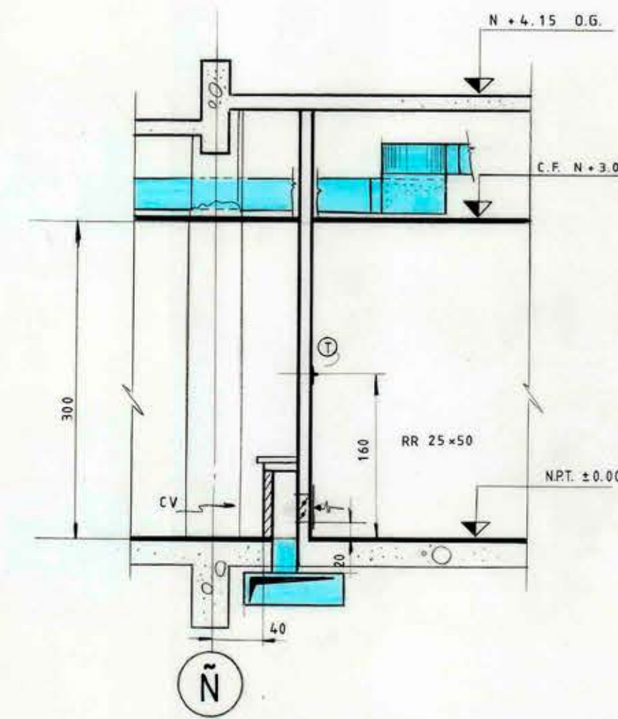
CORTE A-A
