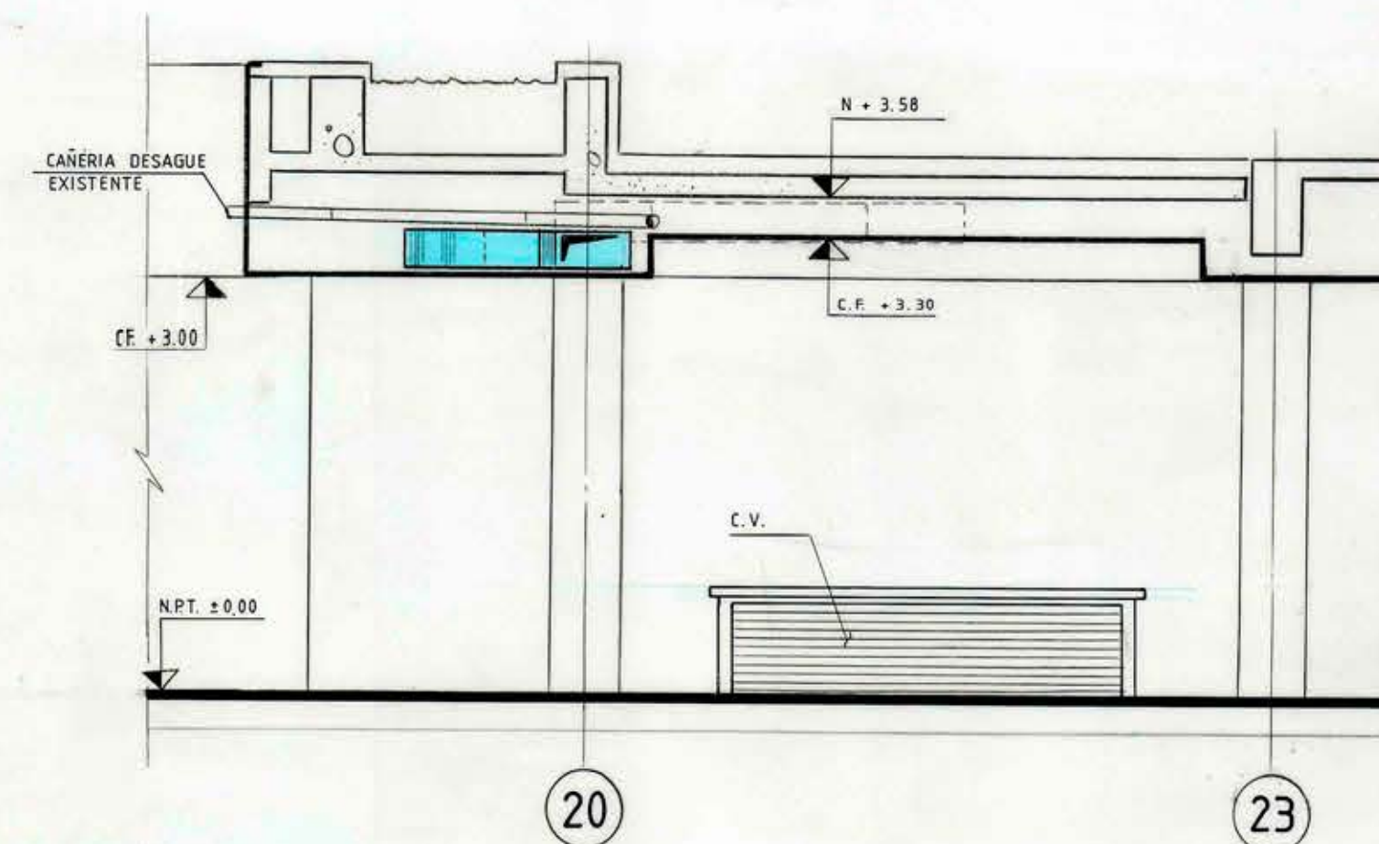
CORTE B-B
