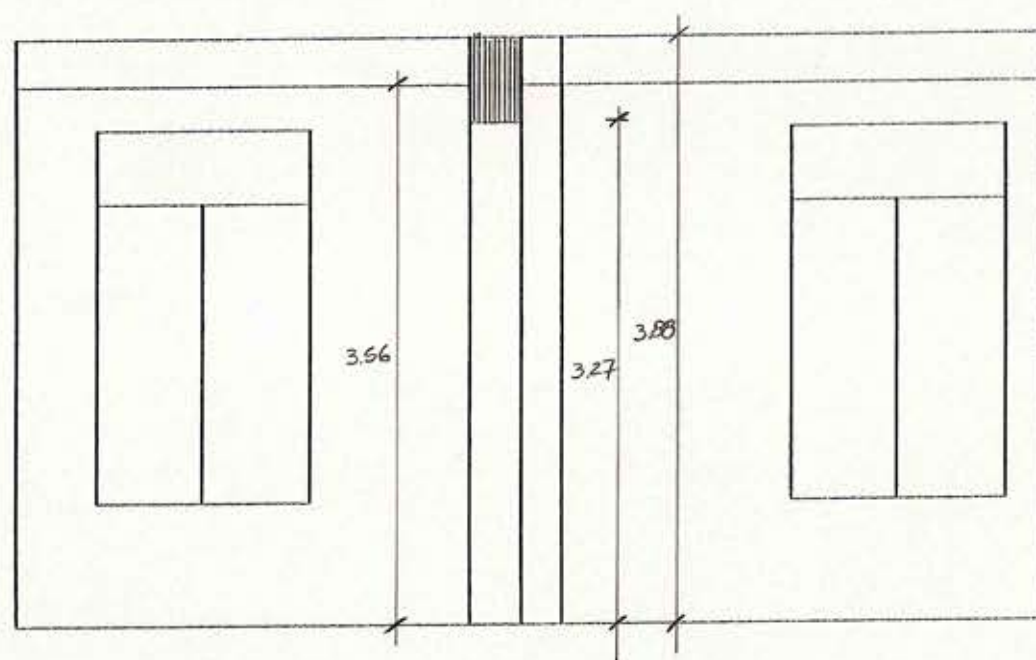
ELEVACION SUR OFICINA SUB SECRETARIO JUSTICIA (ESC. 1:50)
