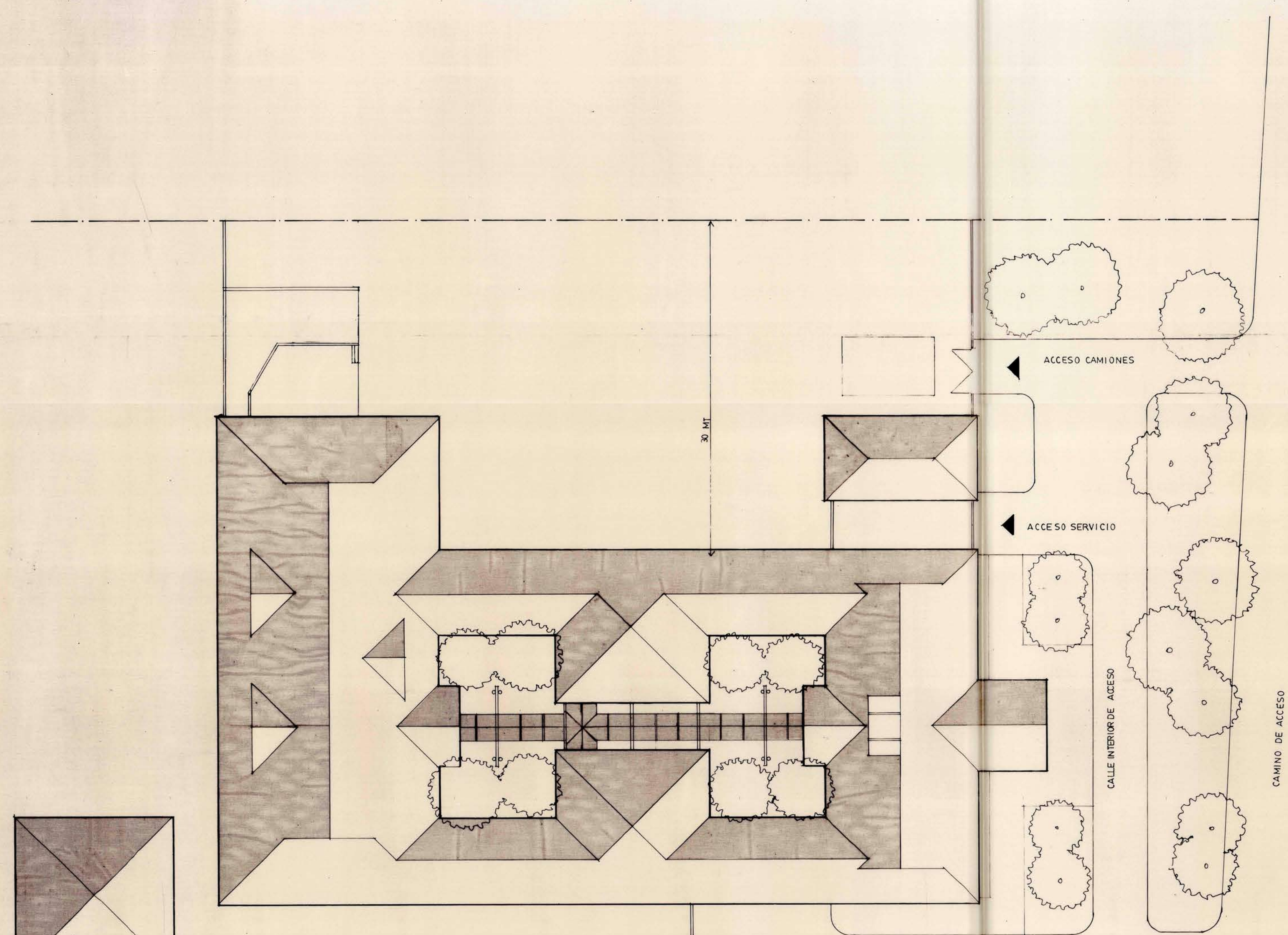
PLANTA DE TECHOS ESC. 1:200 YEMPLAZAMIENTO
