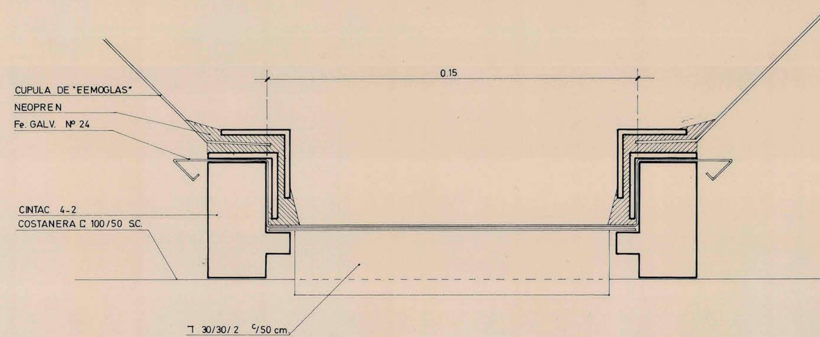
DETALLE 1 ESCALA 1:1
