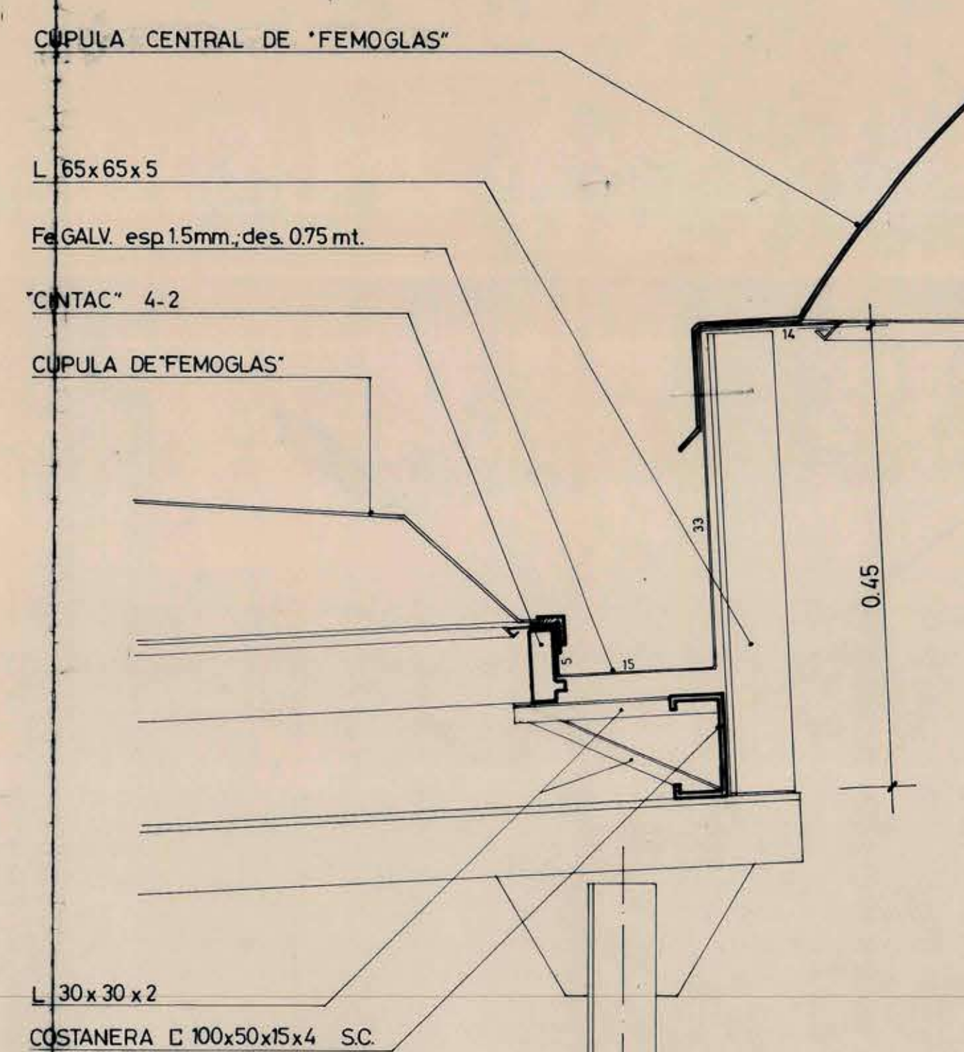
DETALLE 2 ESCALA 1:5
