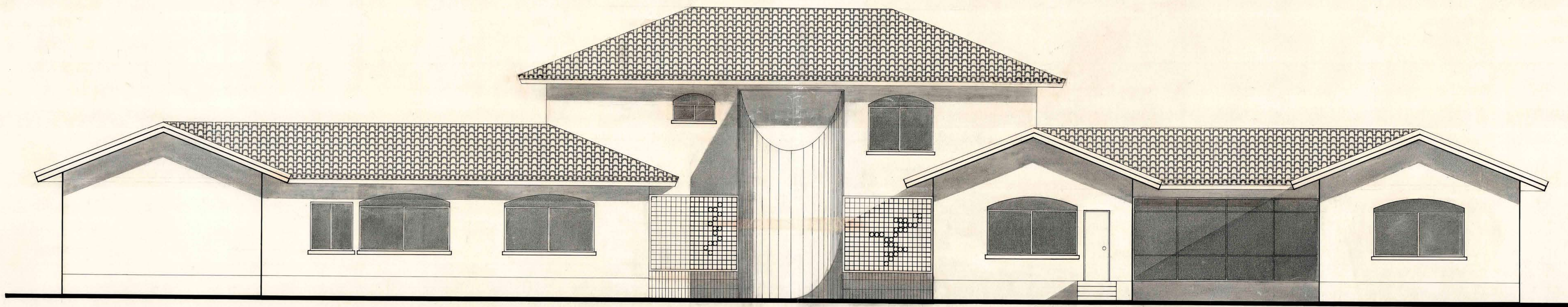
ELEVACION SUR ESCALA 1:50
