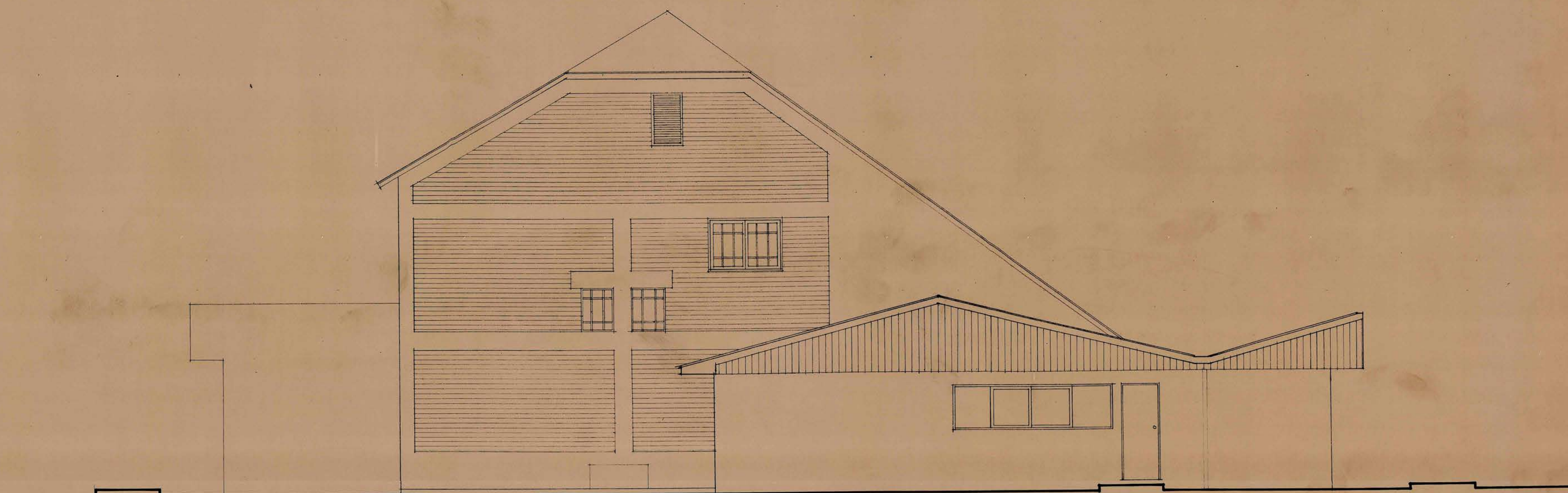
FACHADA ORIENTE Esc. 1:50
