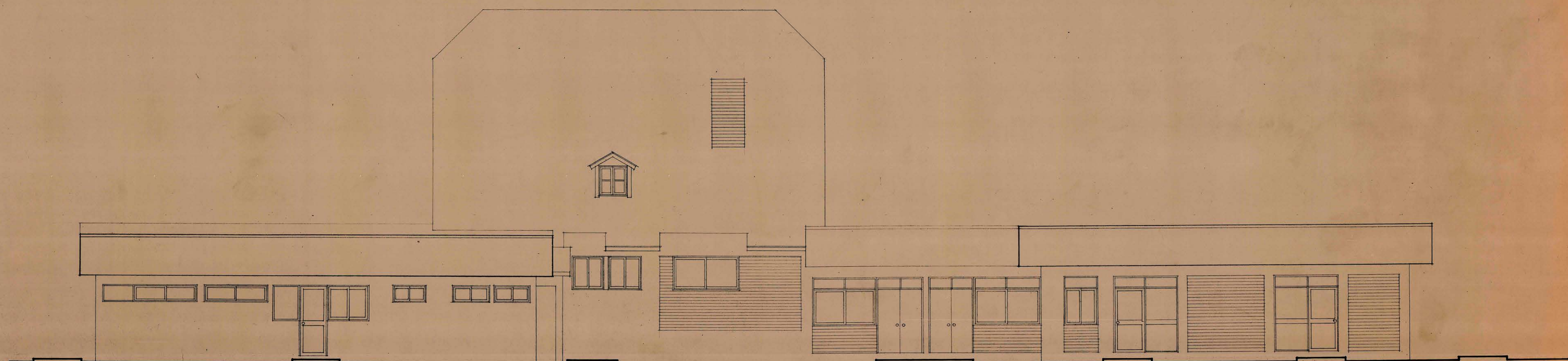
FACHADA SUR E90.1:50
