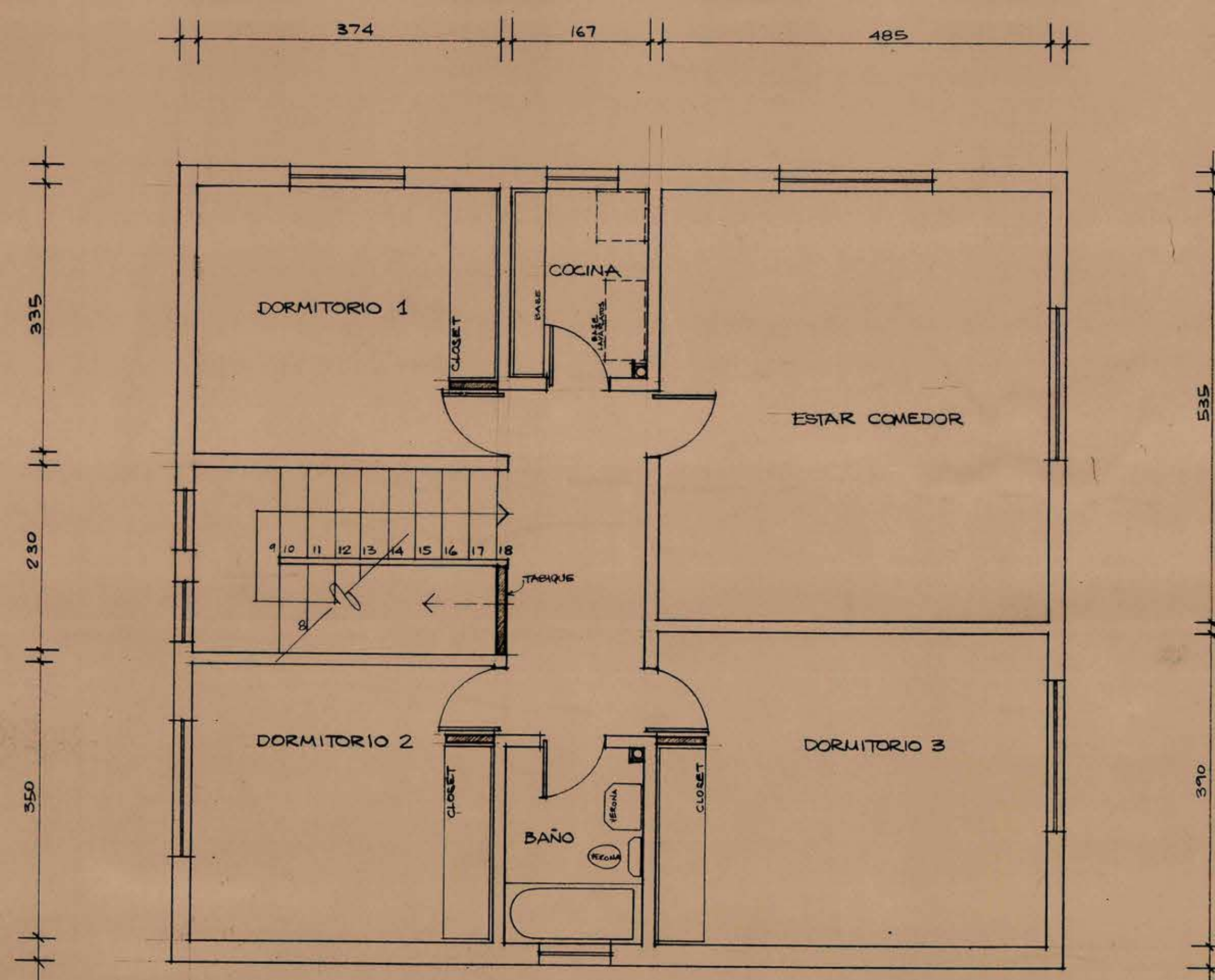
PLANTA 2º PISO ESC. 1:50
