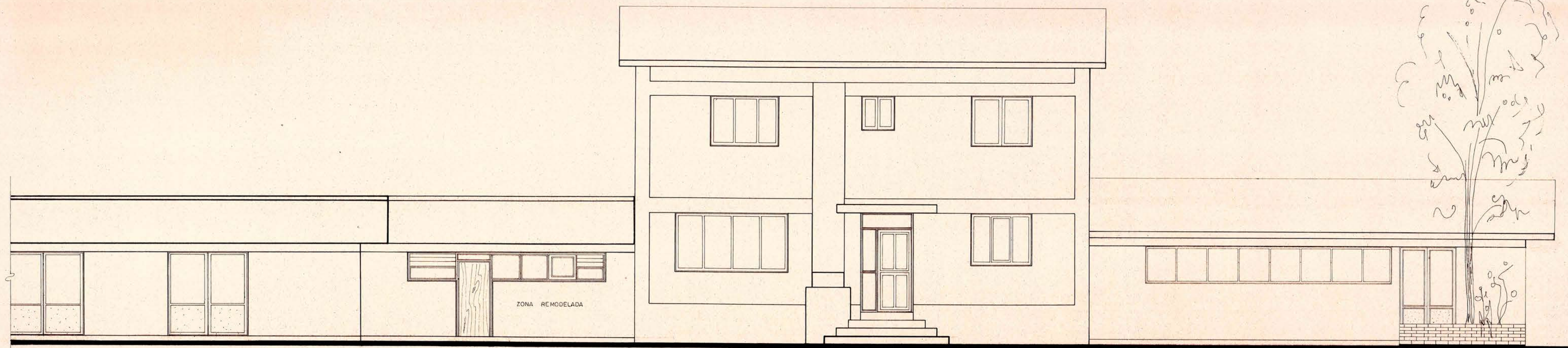
ELEVACION PRINCIPAL
