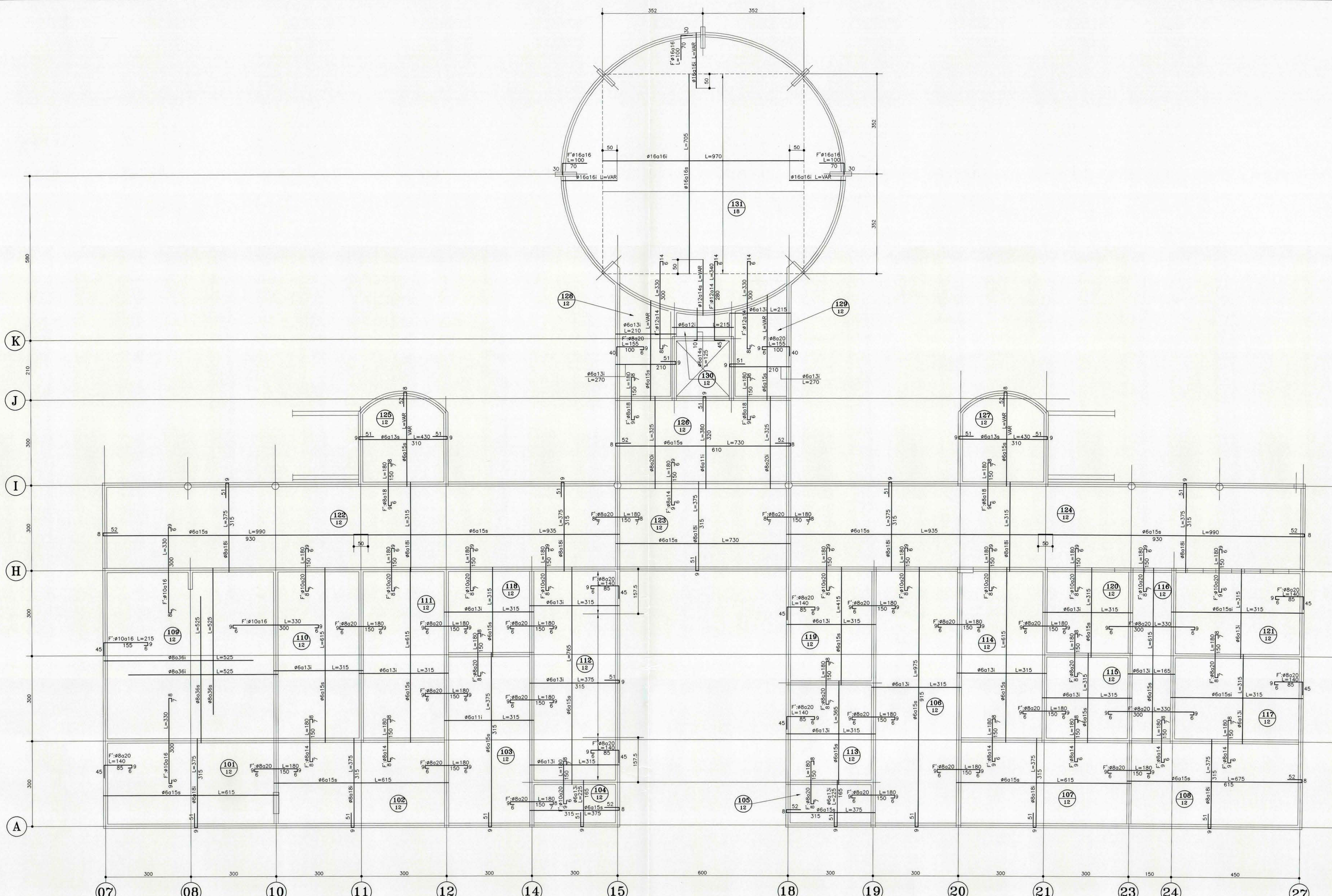
PLANTA ARMADURA DE LOSAS CIELO 1° ESC. 1:50
