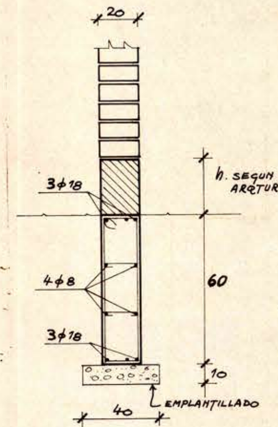
SECC. VIGAS FUND. EN GÁRDONES SIN LOSAS
