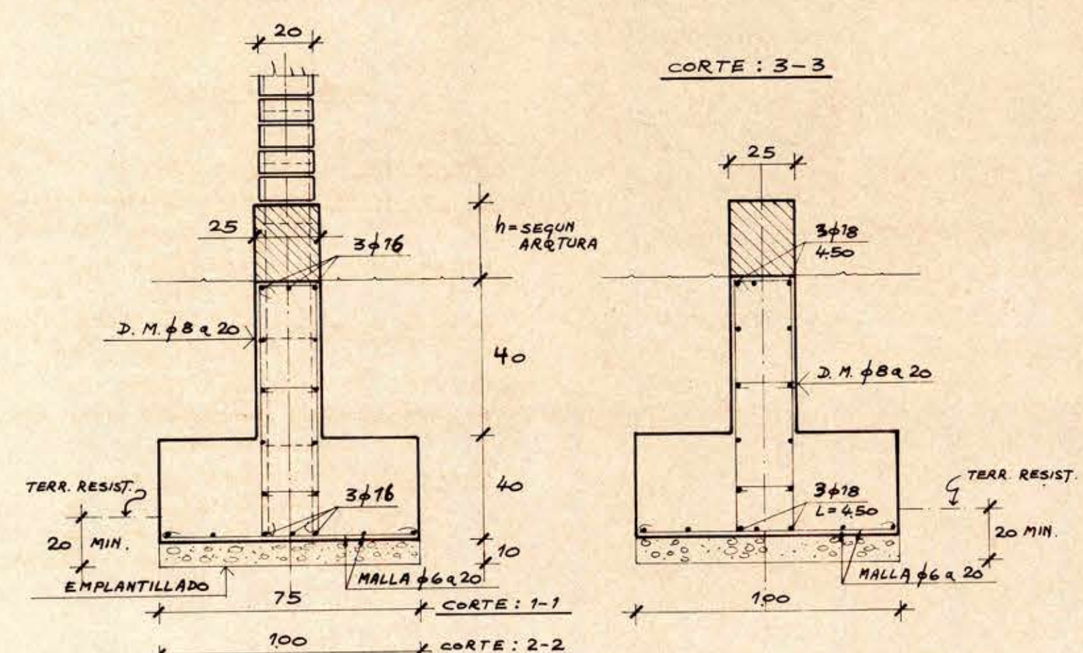
CORTES: 1-1 y 2-2
