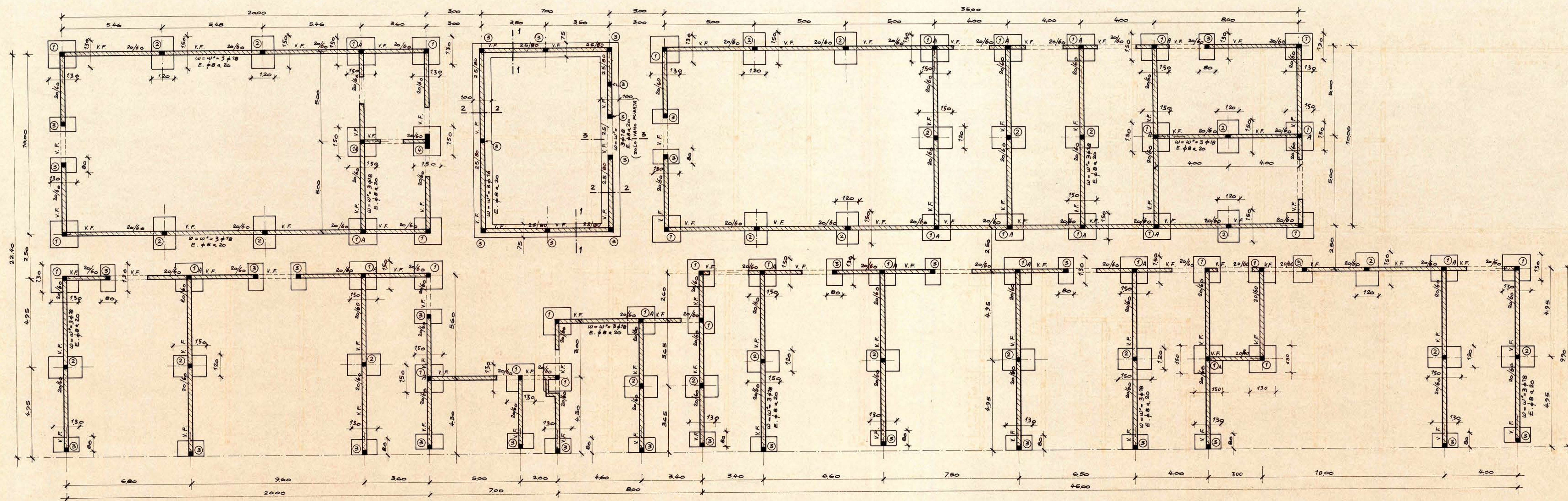
PLANTA DE FUNDACIONES.
