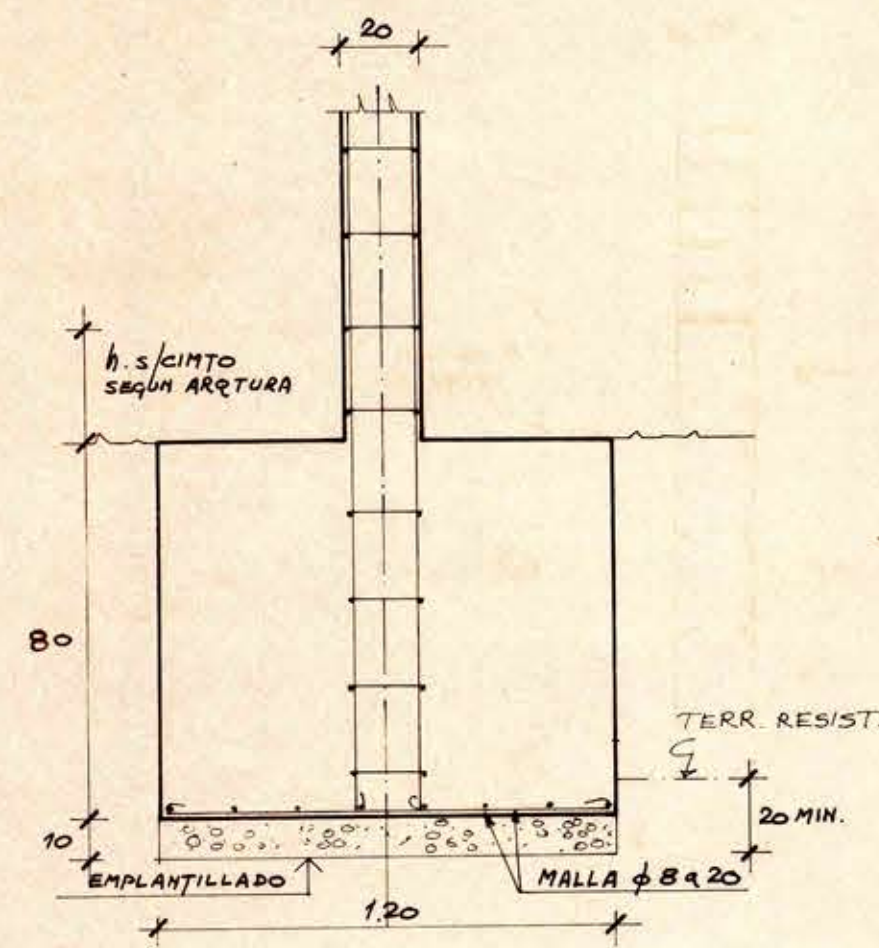
FUND. DADOS PIL. 2
