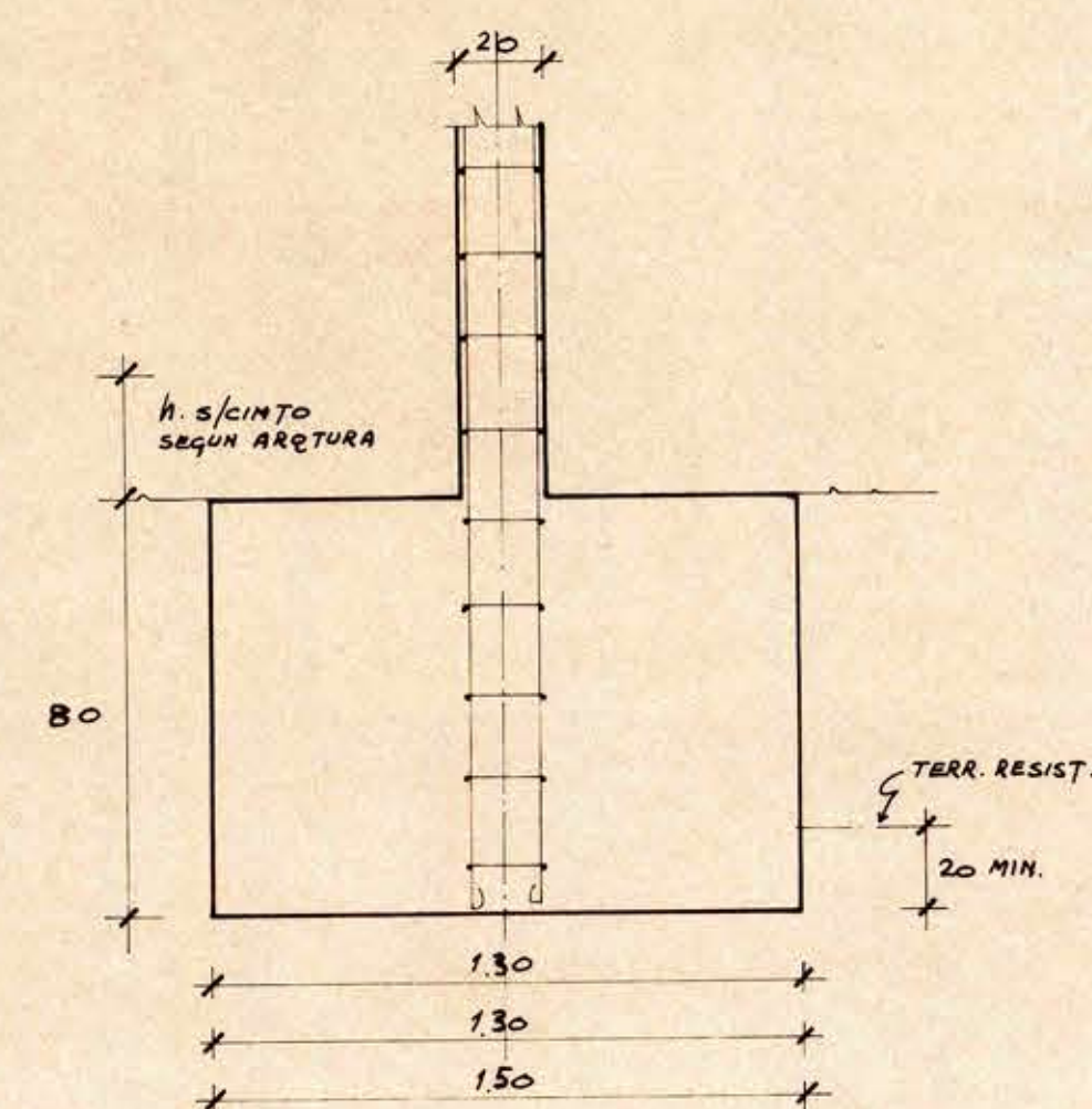
FUND. DADOS PILARES: 1-10 y 11-14
